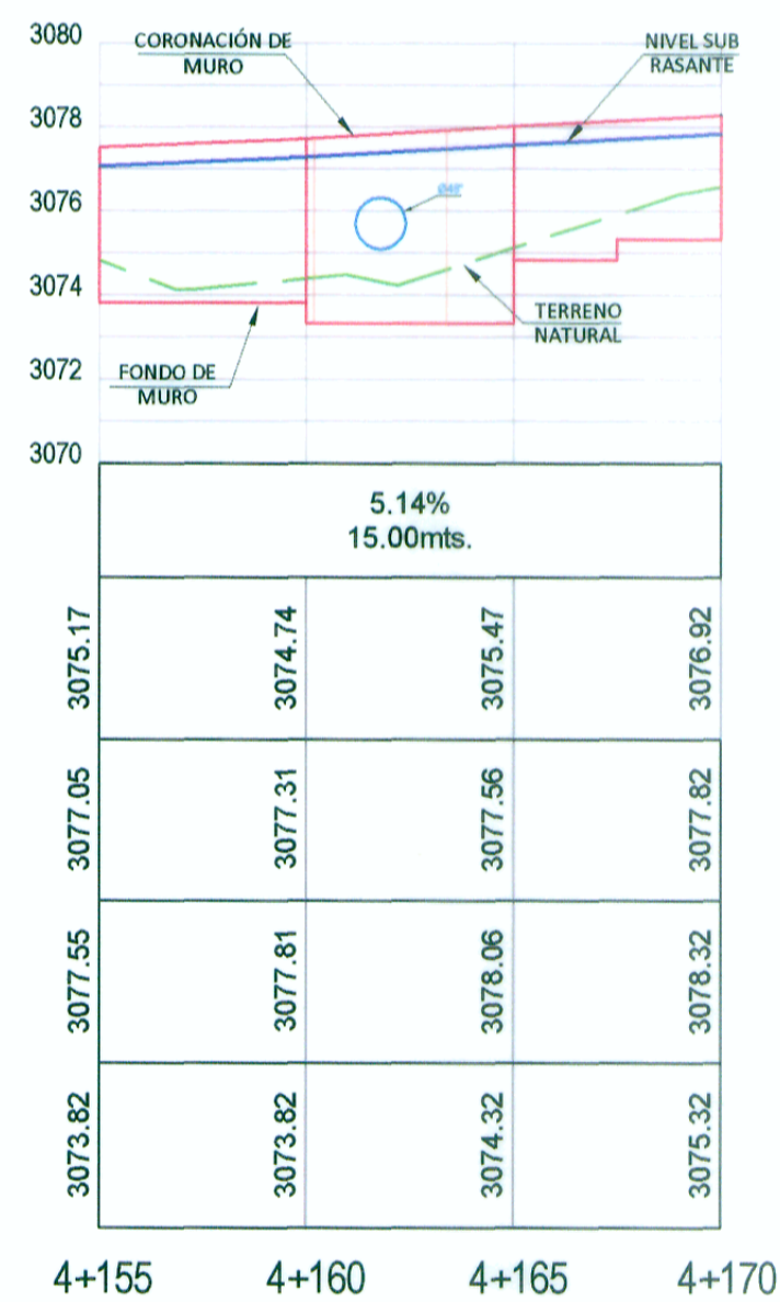
PERFIL LONGITUDINAL
