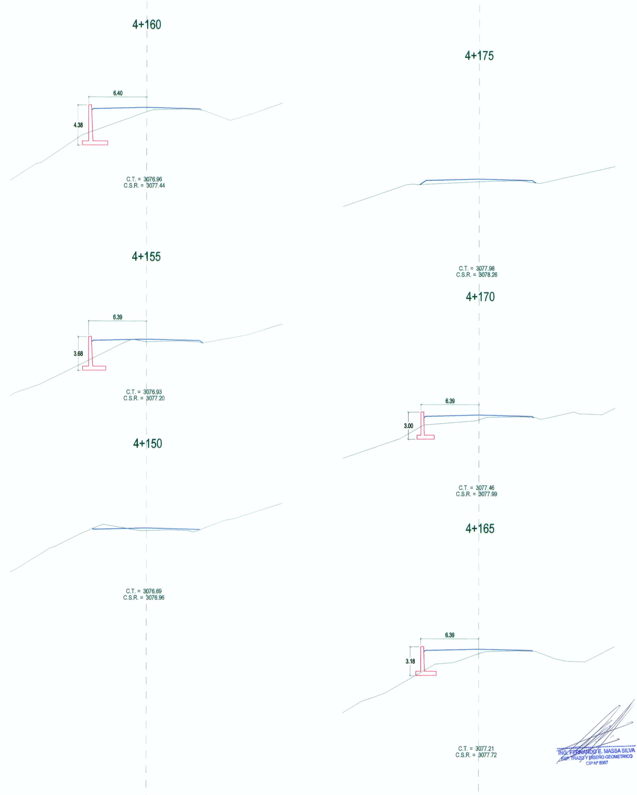
SECCIONES TRANSVERSALES
