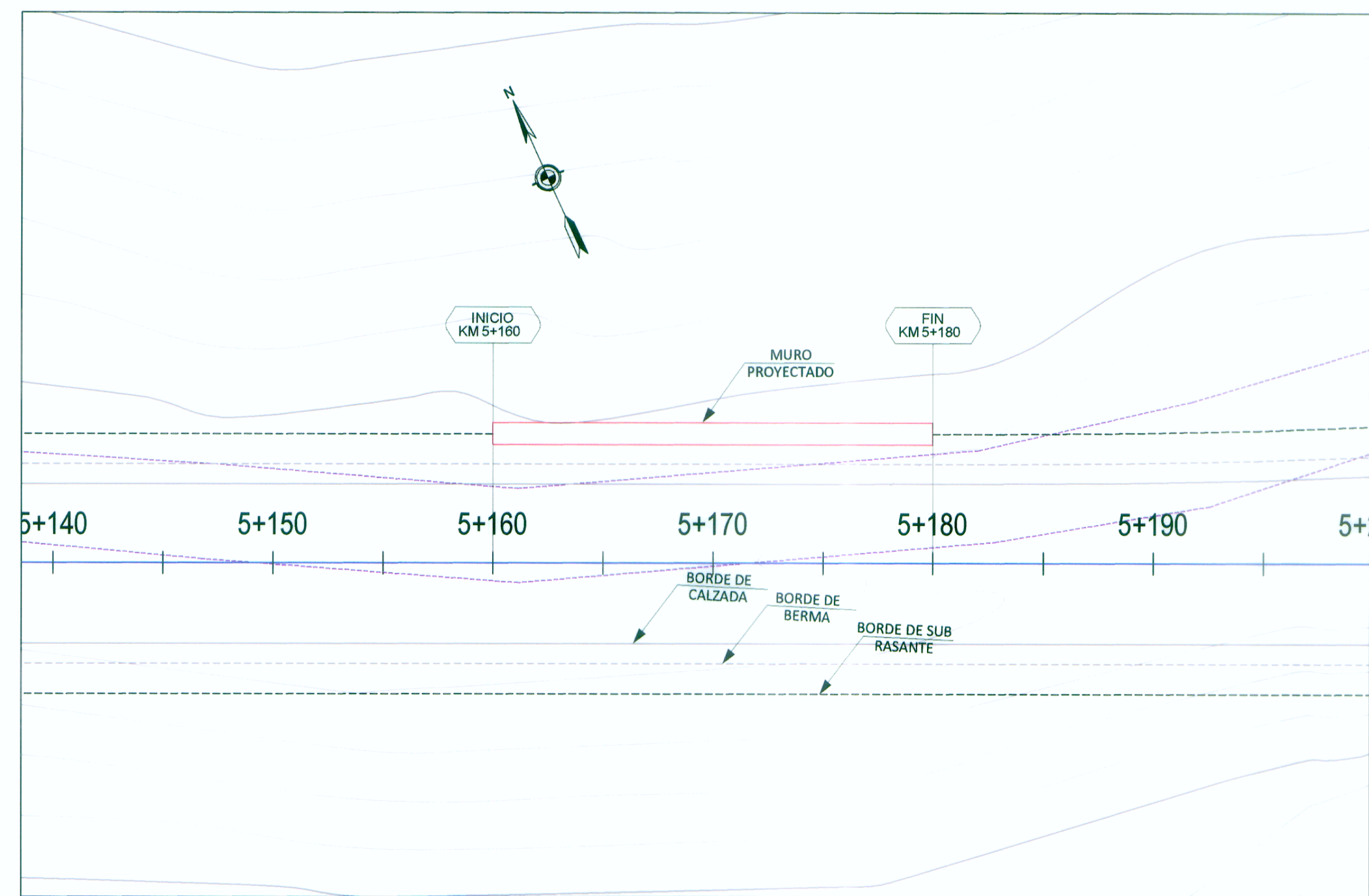
PLANTA
