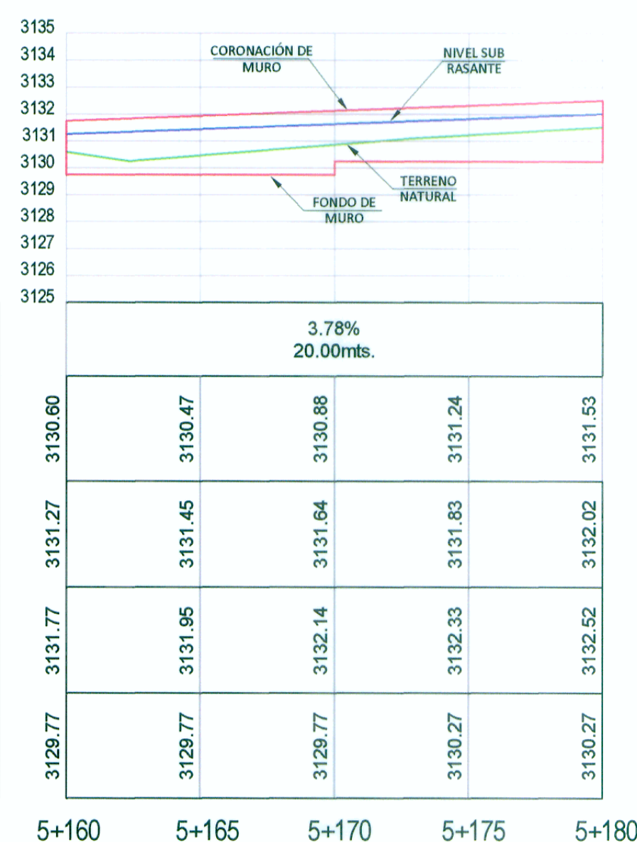
PERFIL LONGITUDINAL
