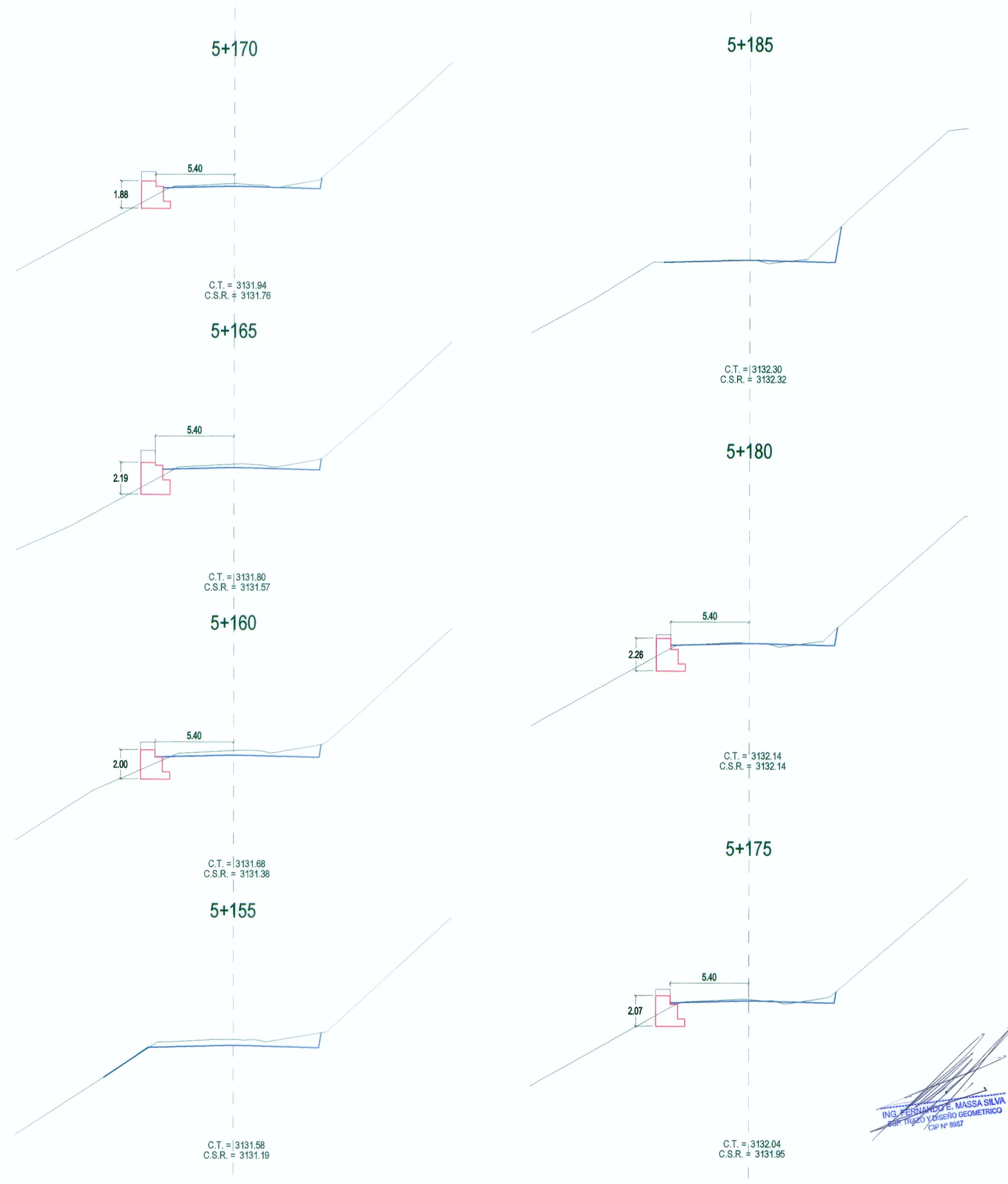
SECCIONES TRANSVERSALES
