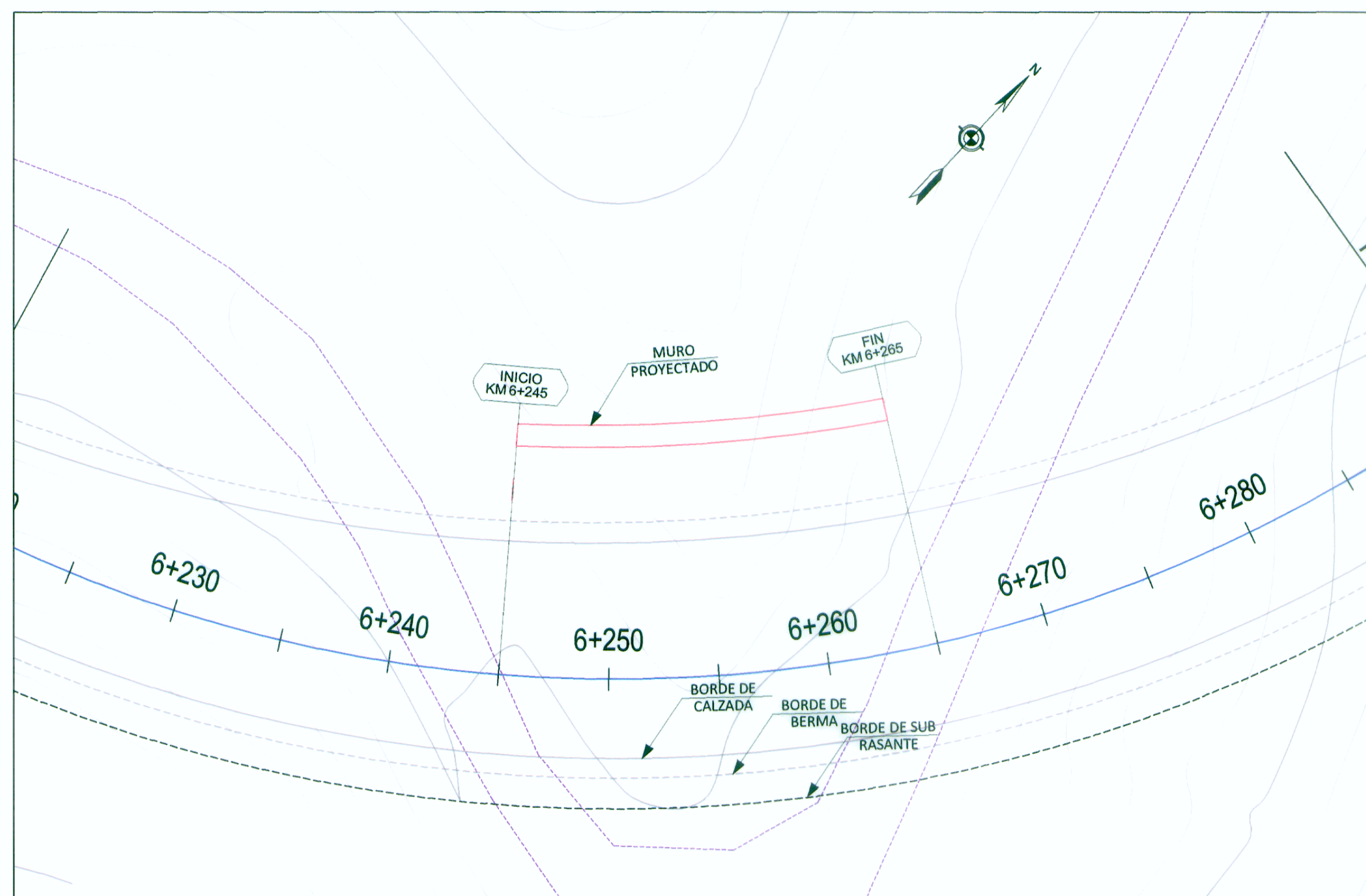
PLANTA
