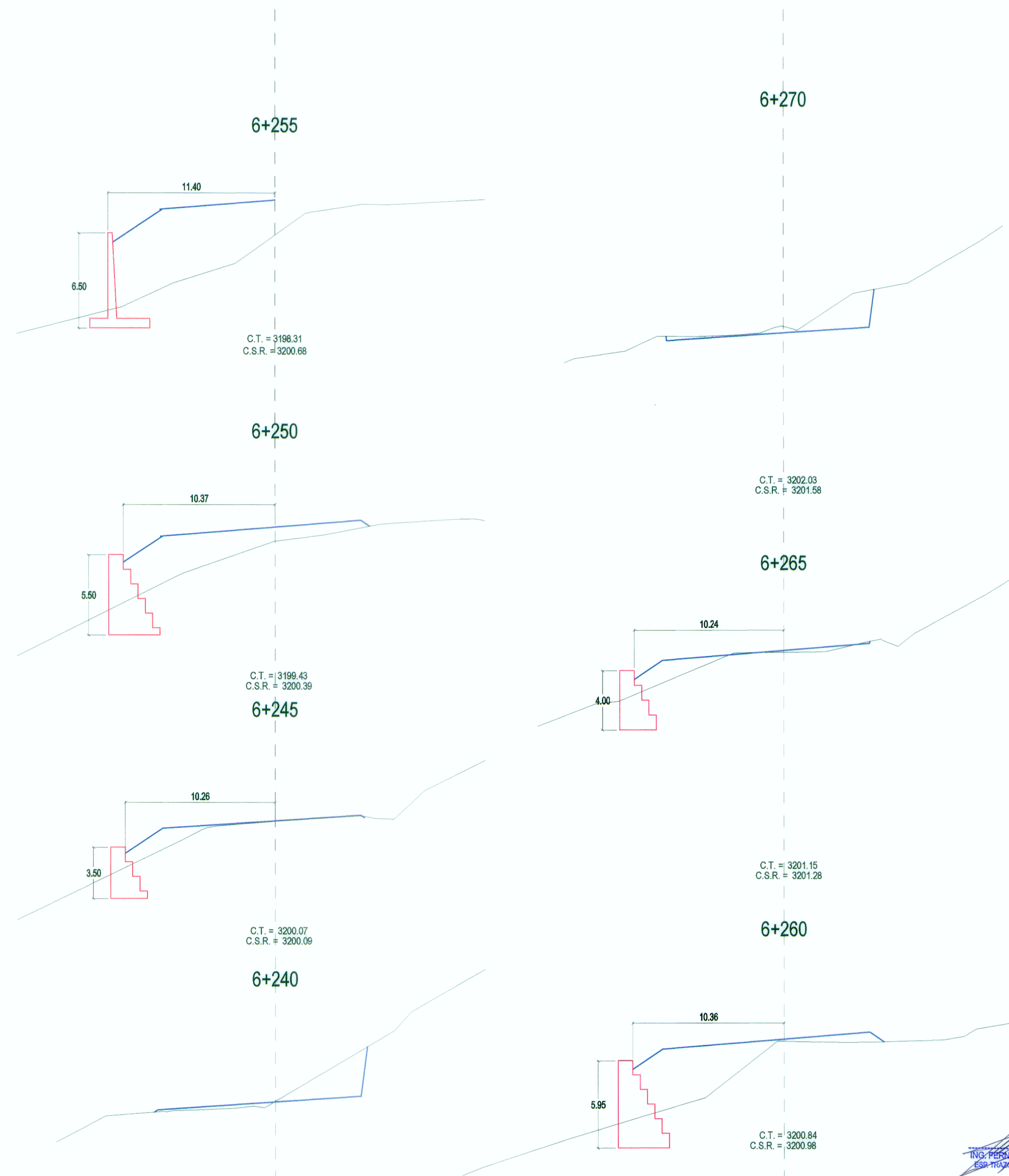
SECCIONES TRANSVERSALES
