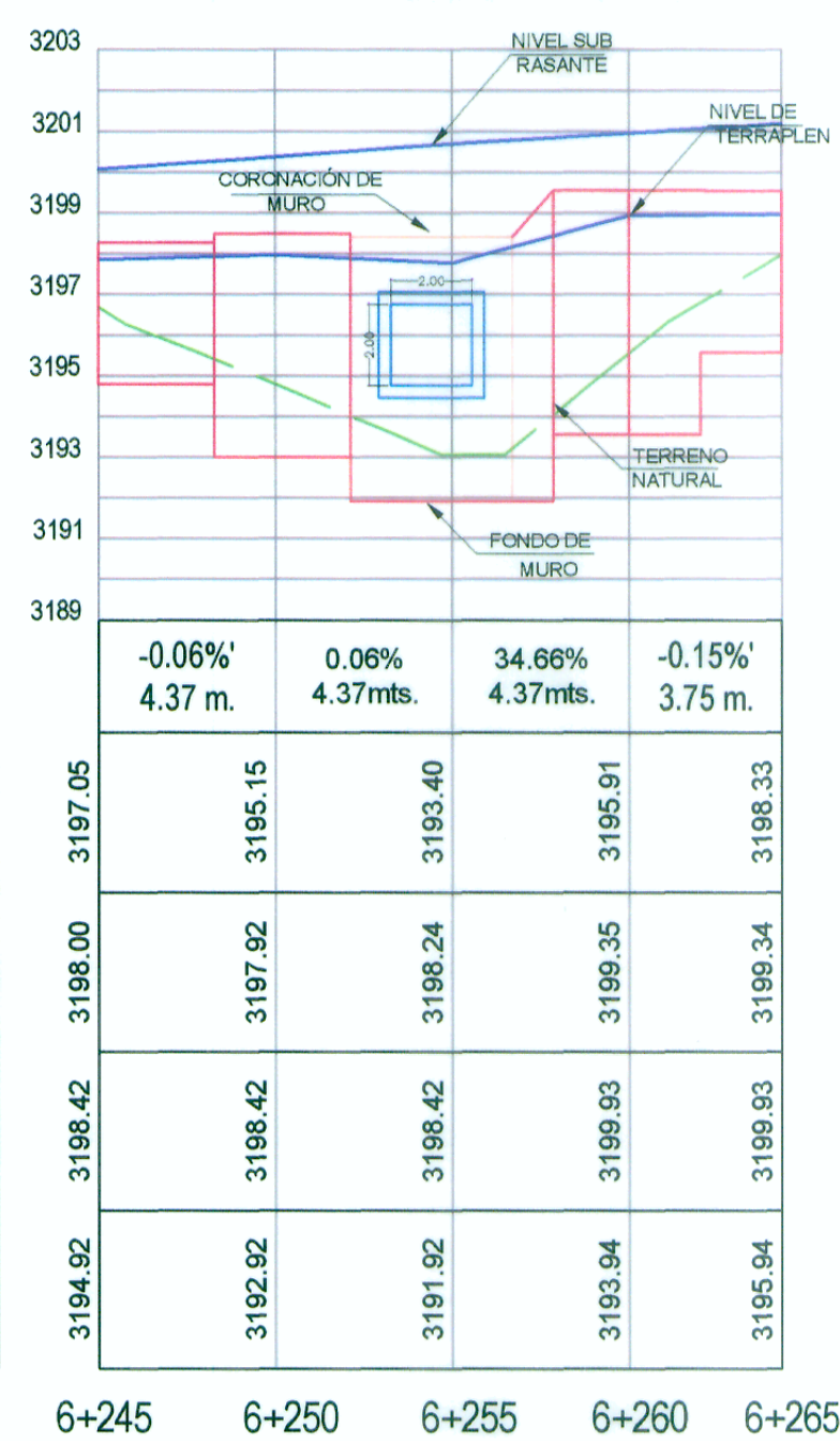
PERFIL LONGITUDINAL
