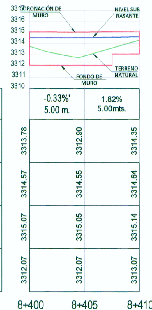
PERFIL LONGITUDINAL
