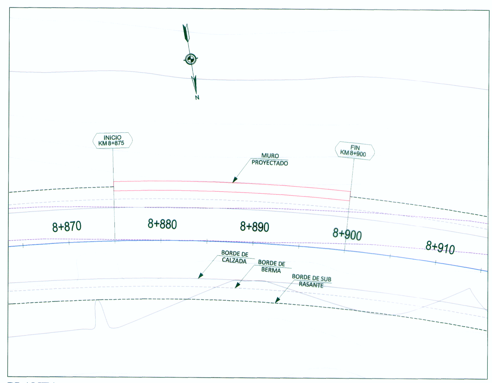
PLANTA
