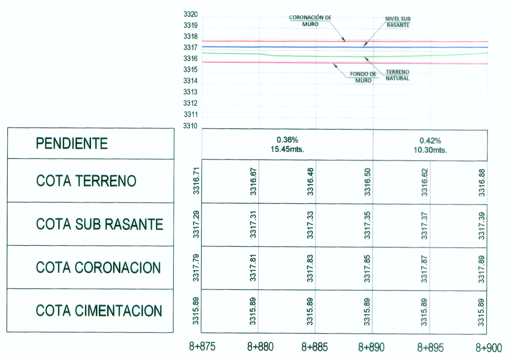
PERFIL LONGITUDINAL
