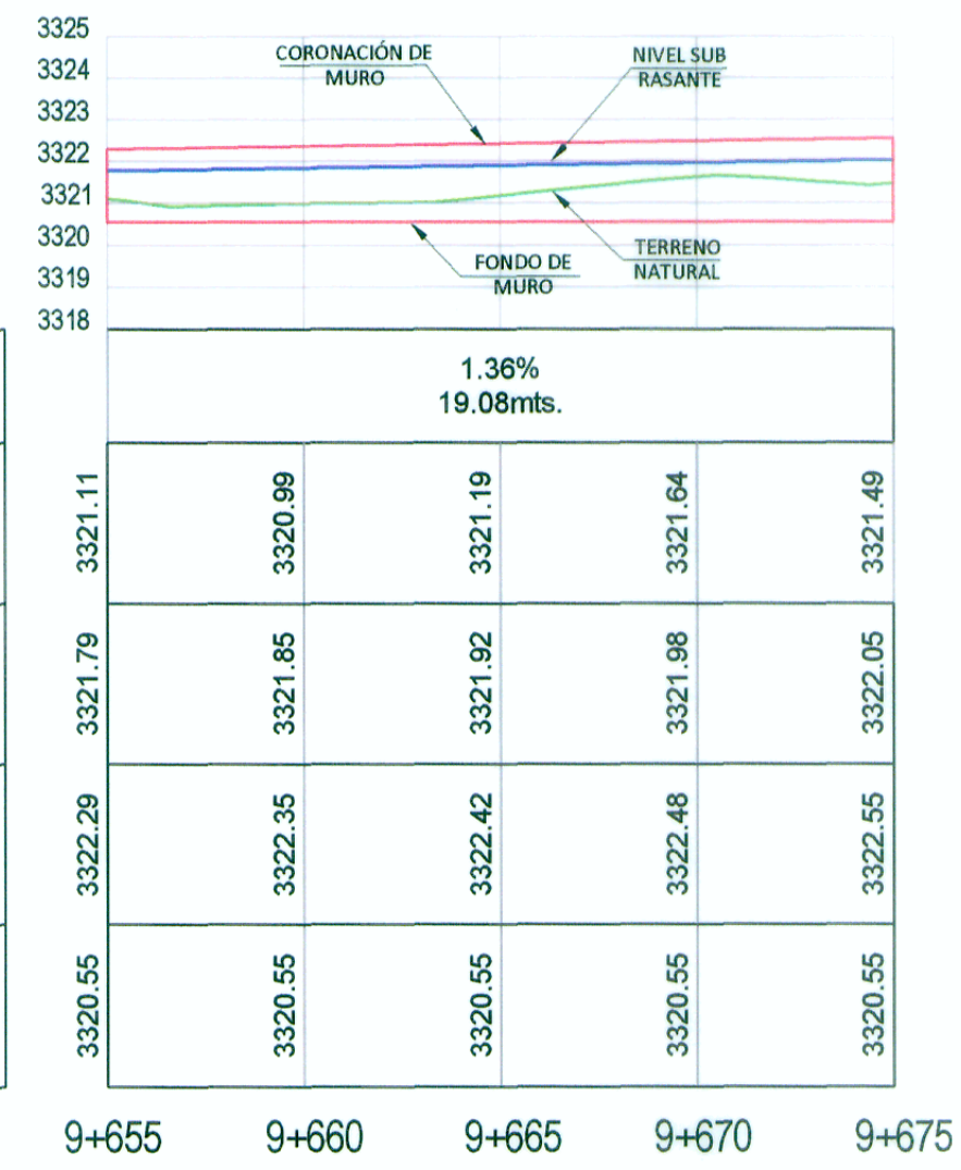
PERFIL LONGITUDINAL
