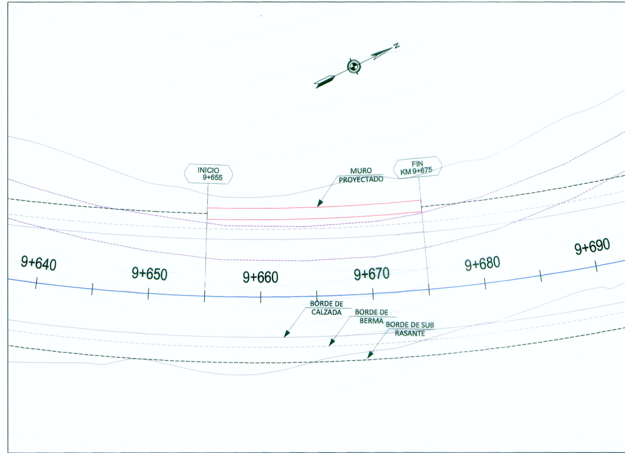
PLANTA
