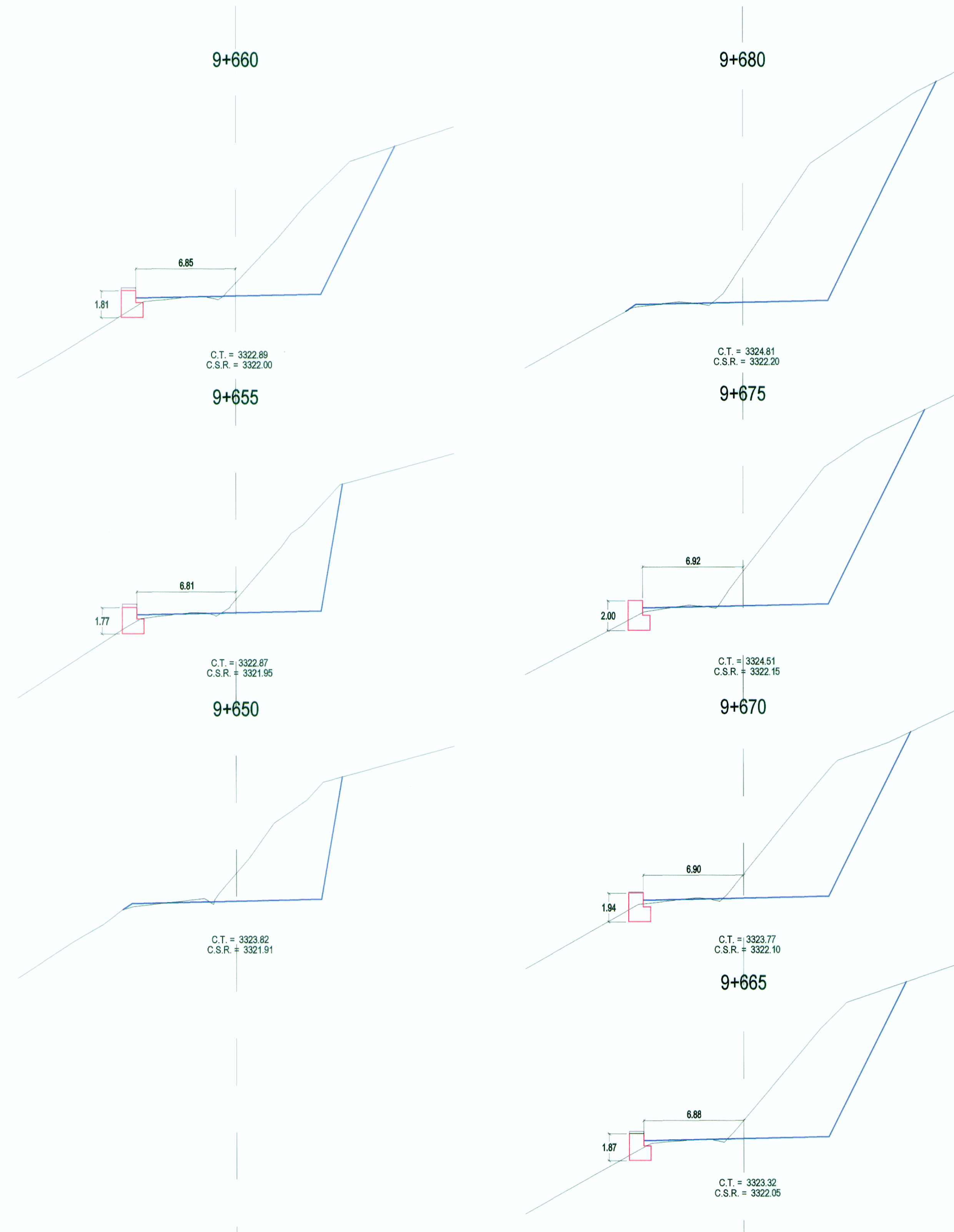
SECCIONES TRANSVERSALES
