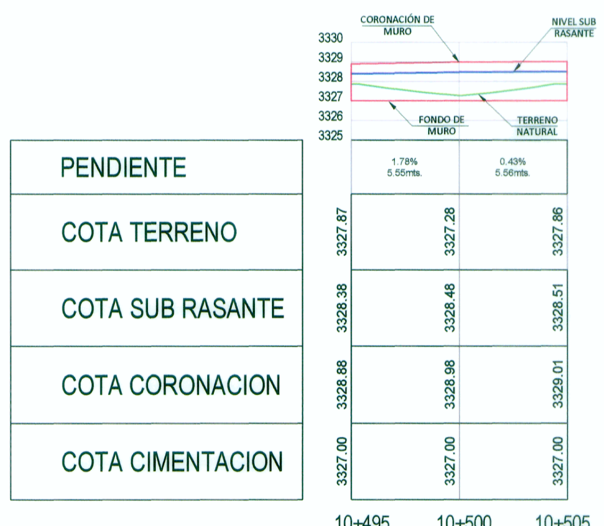
PERFIL LONGITUDINAL
