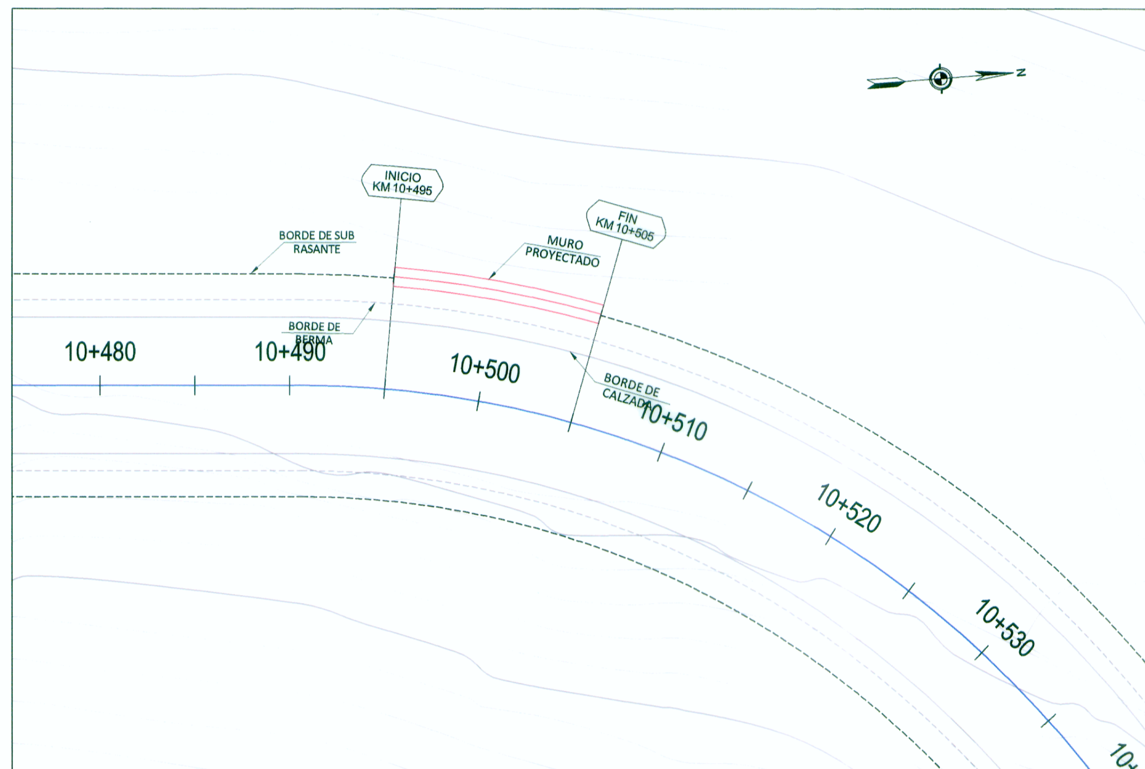
PLANTA
