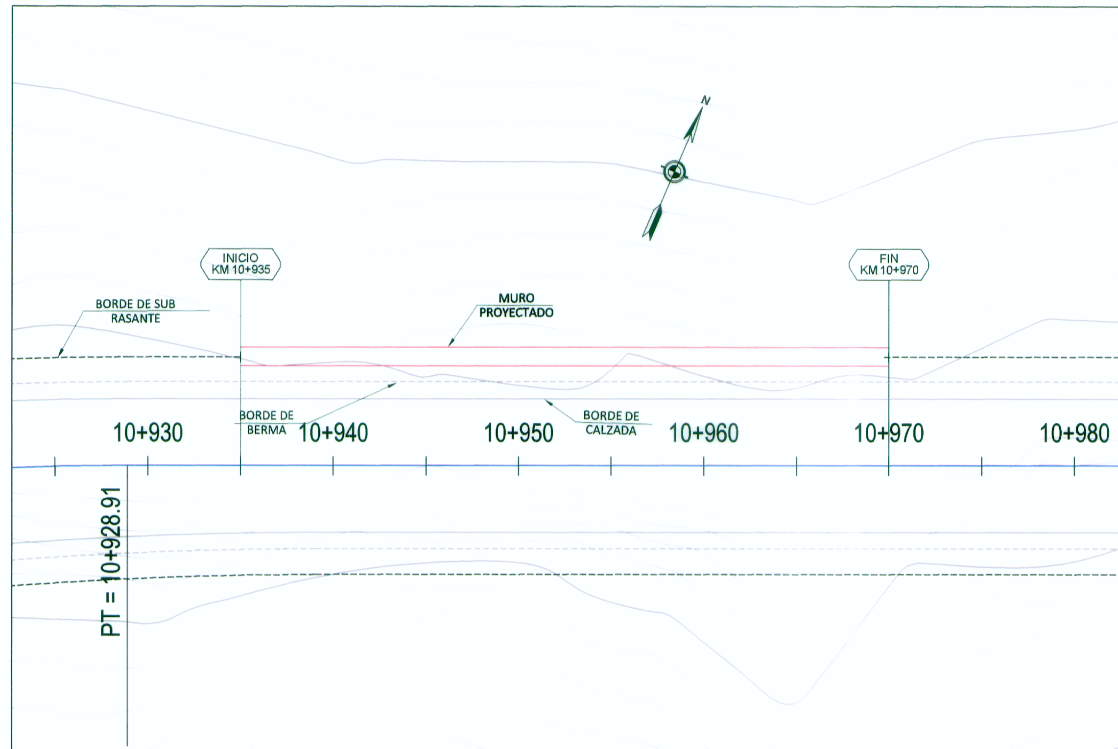
PLANTA
