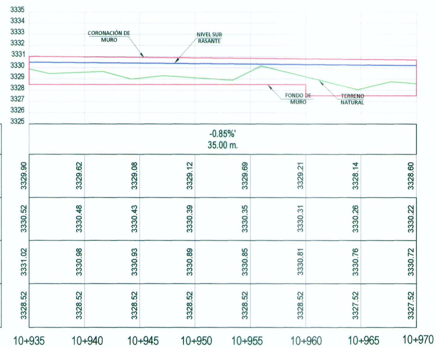
PERFIL LONGITUDINAL
