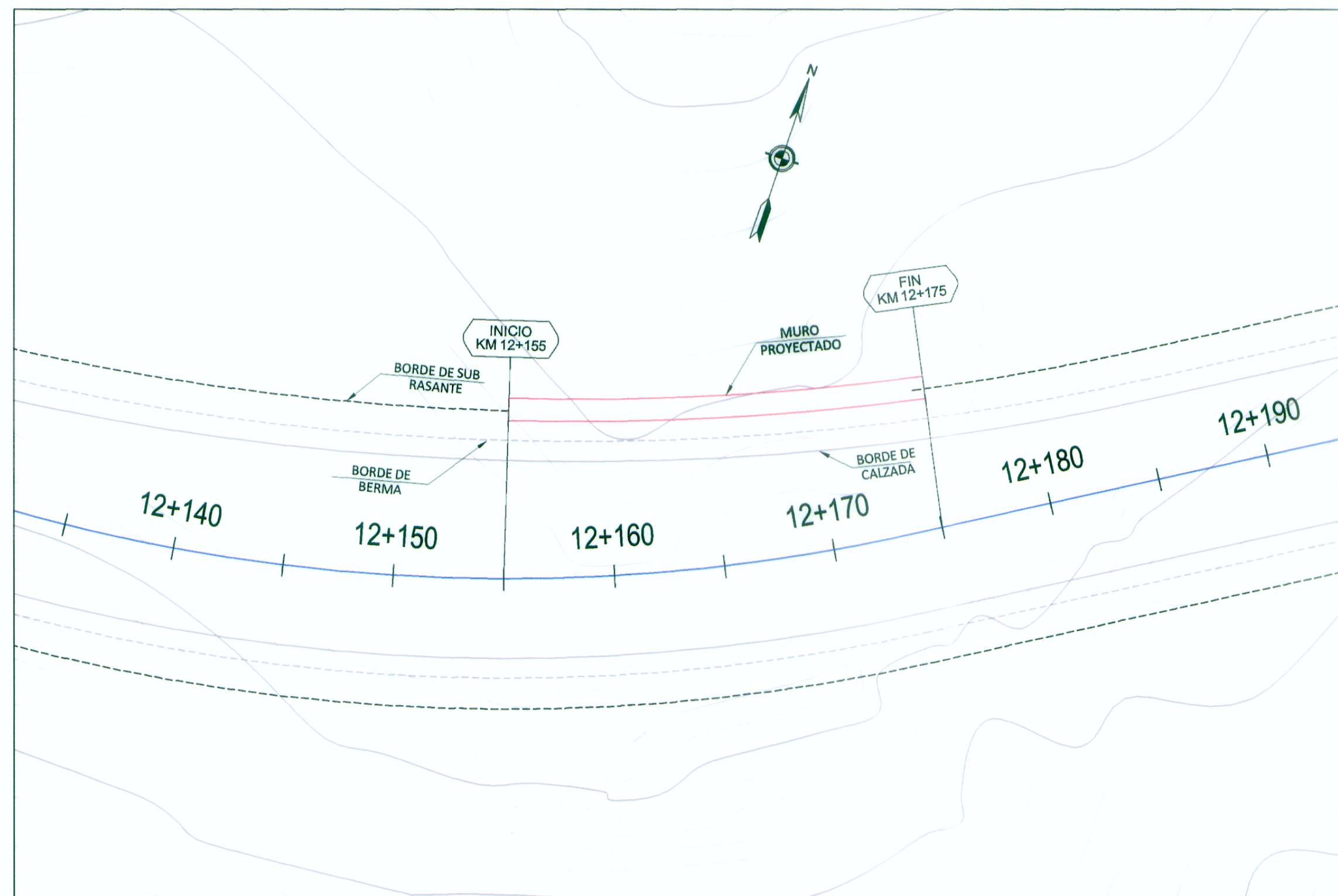
PLANTA
