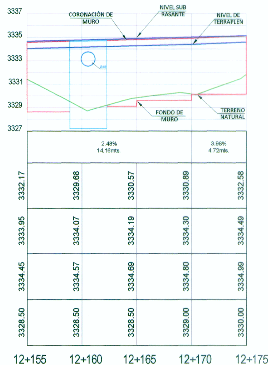
PERFIL LONGITUDINAL
