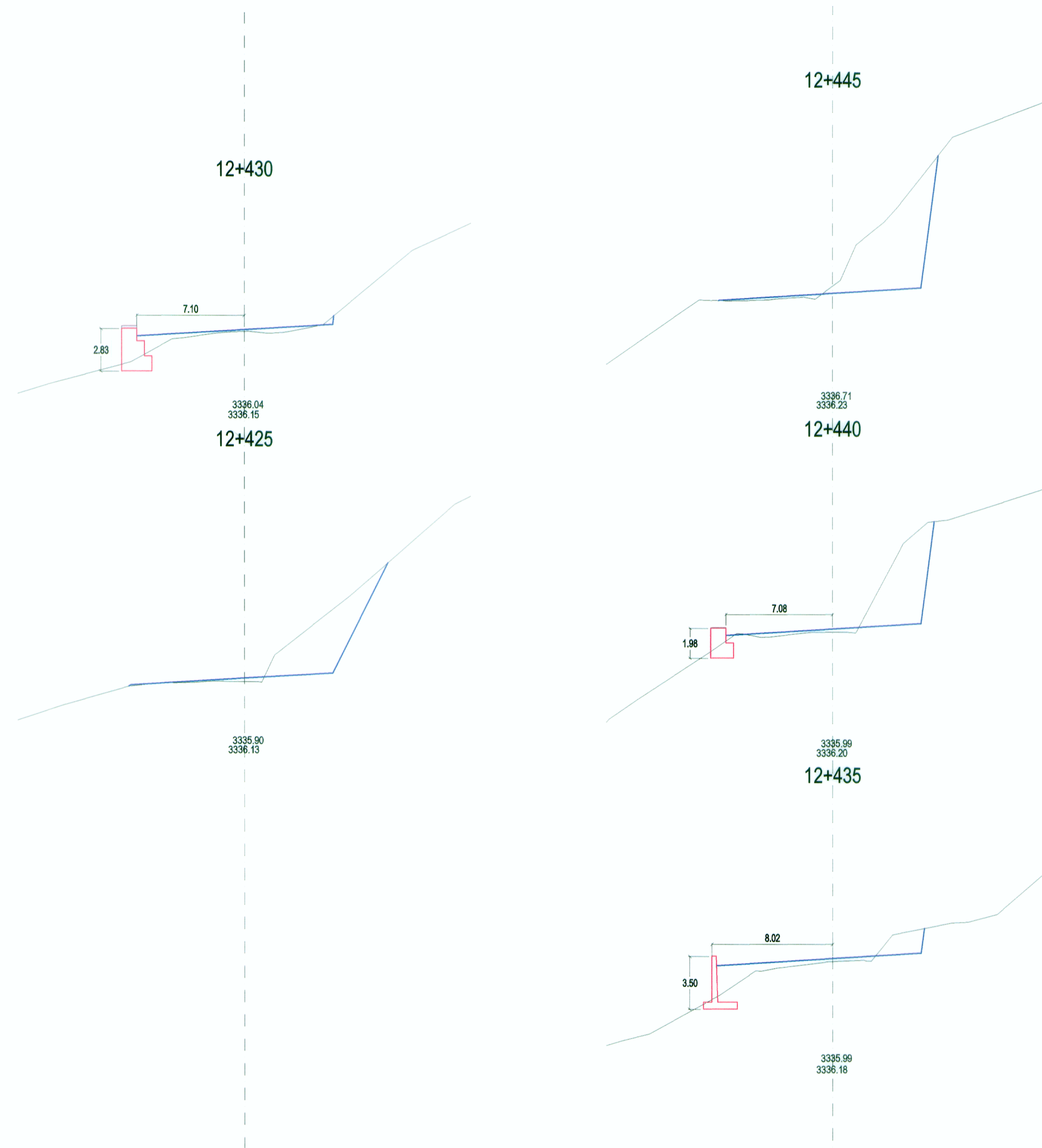
SECCIONES TRANSVERSALES
