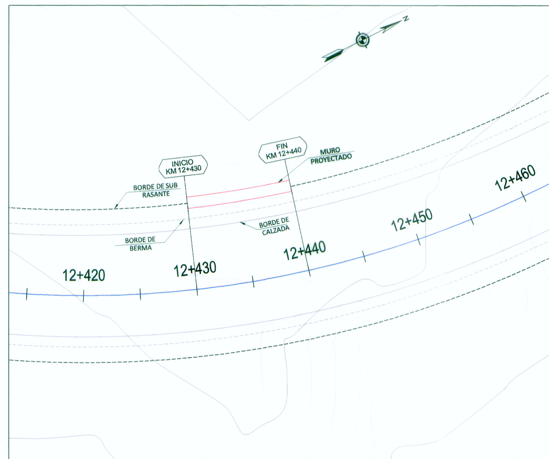
PLANTA
