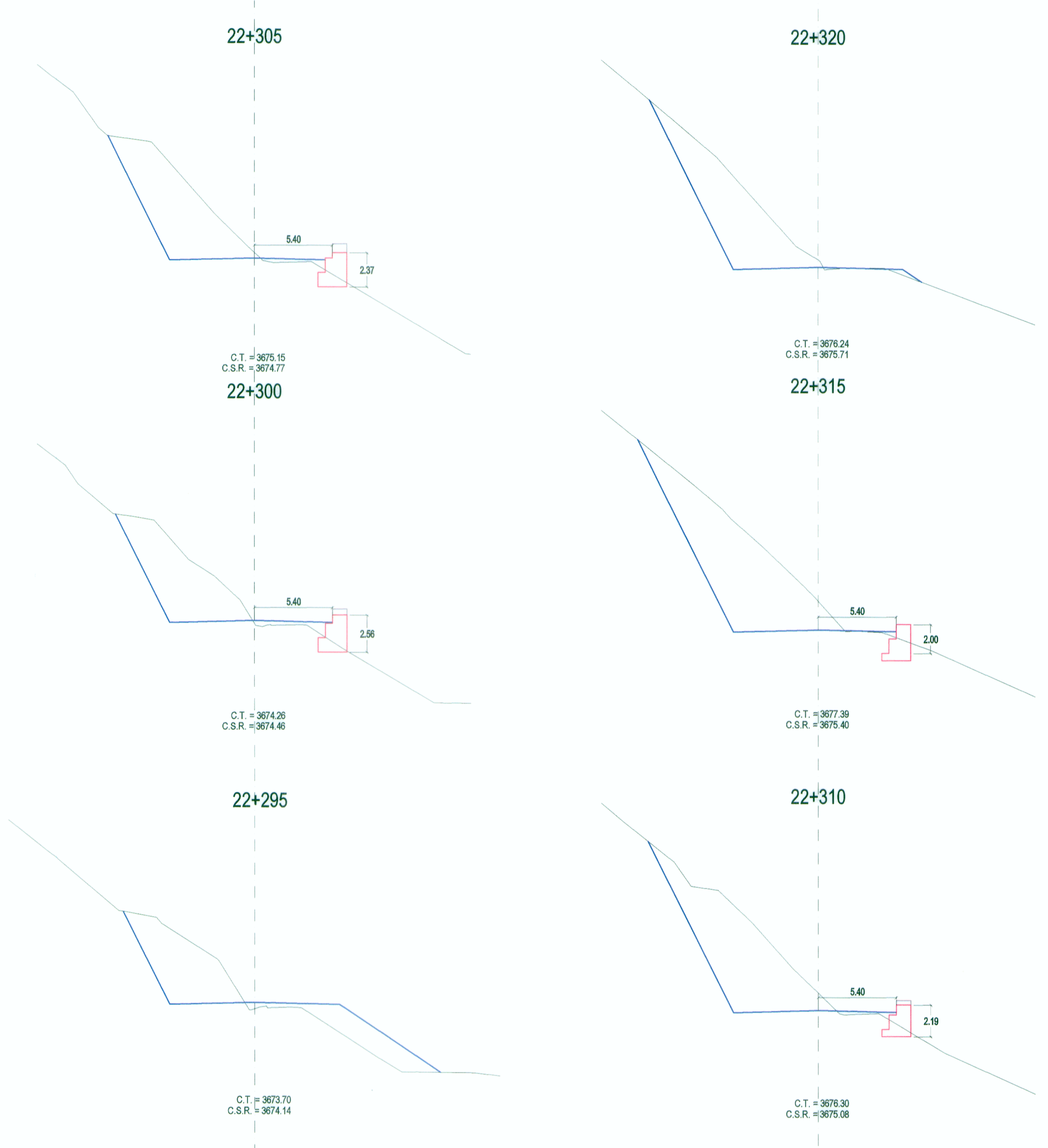
SECCIONES TRANSVERSALES
