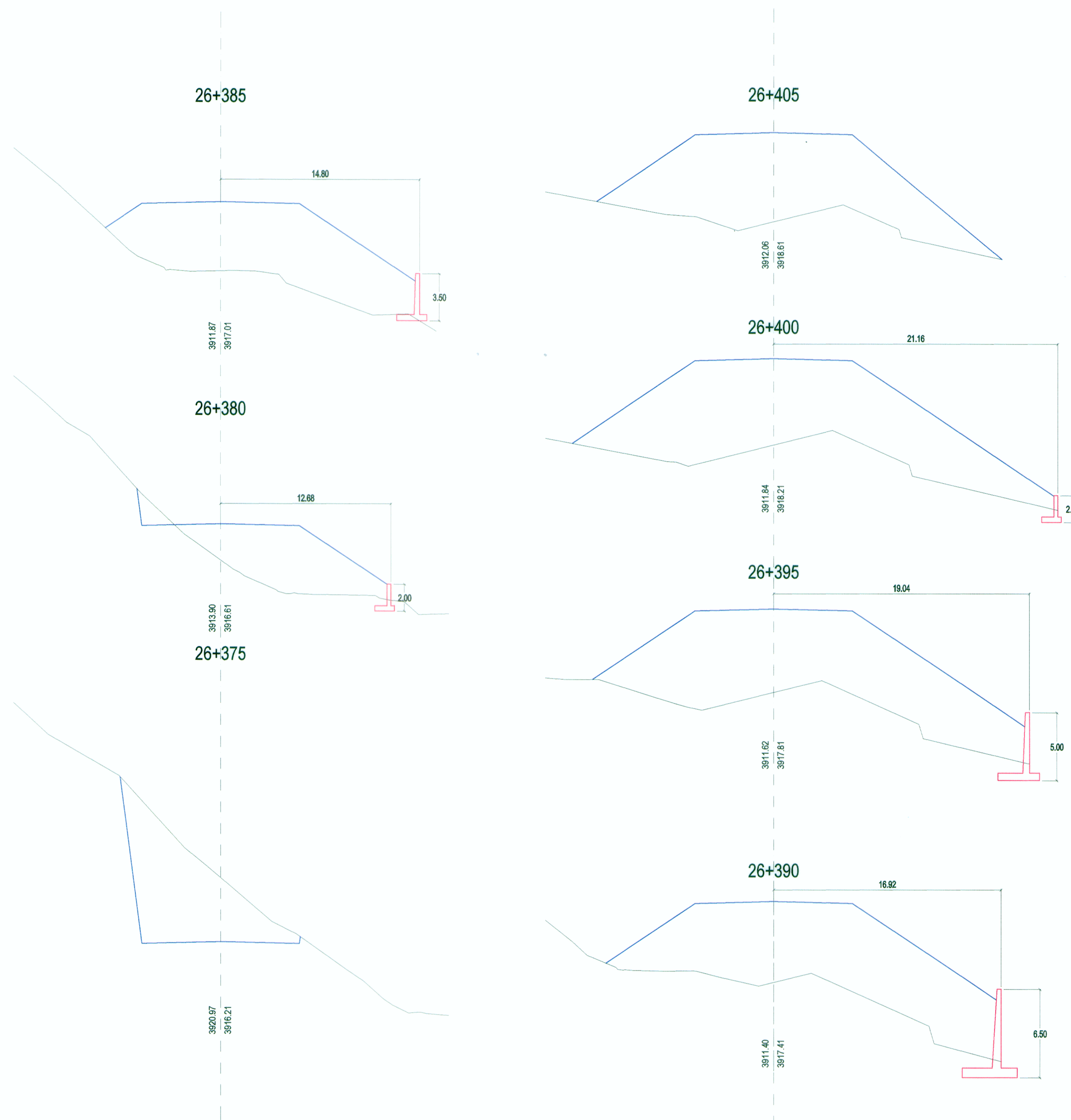
SECCIONES TRANSVERSALES
