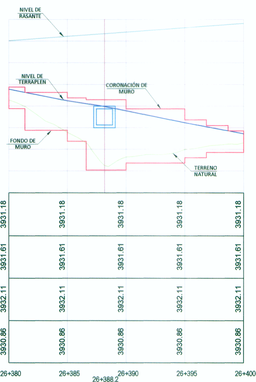
Muro 26+380 - 26+400
