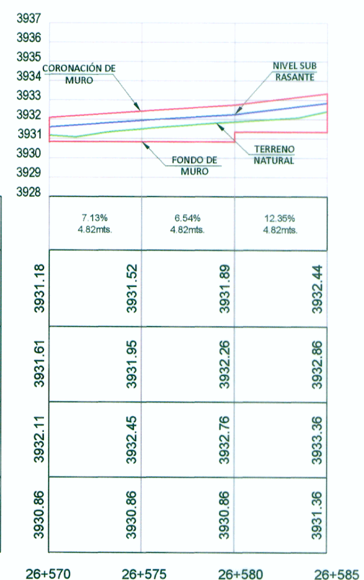
PERFIL LONGITUDINAL
