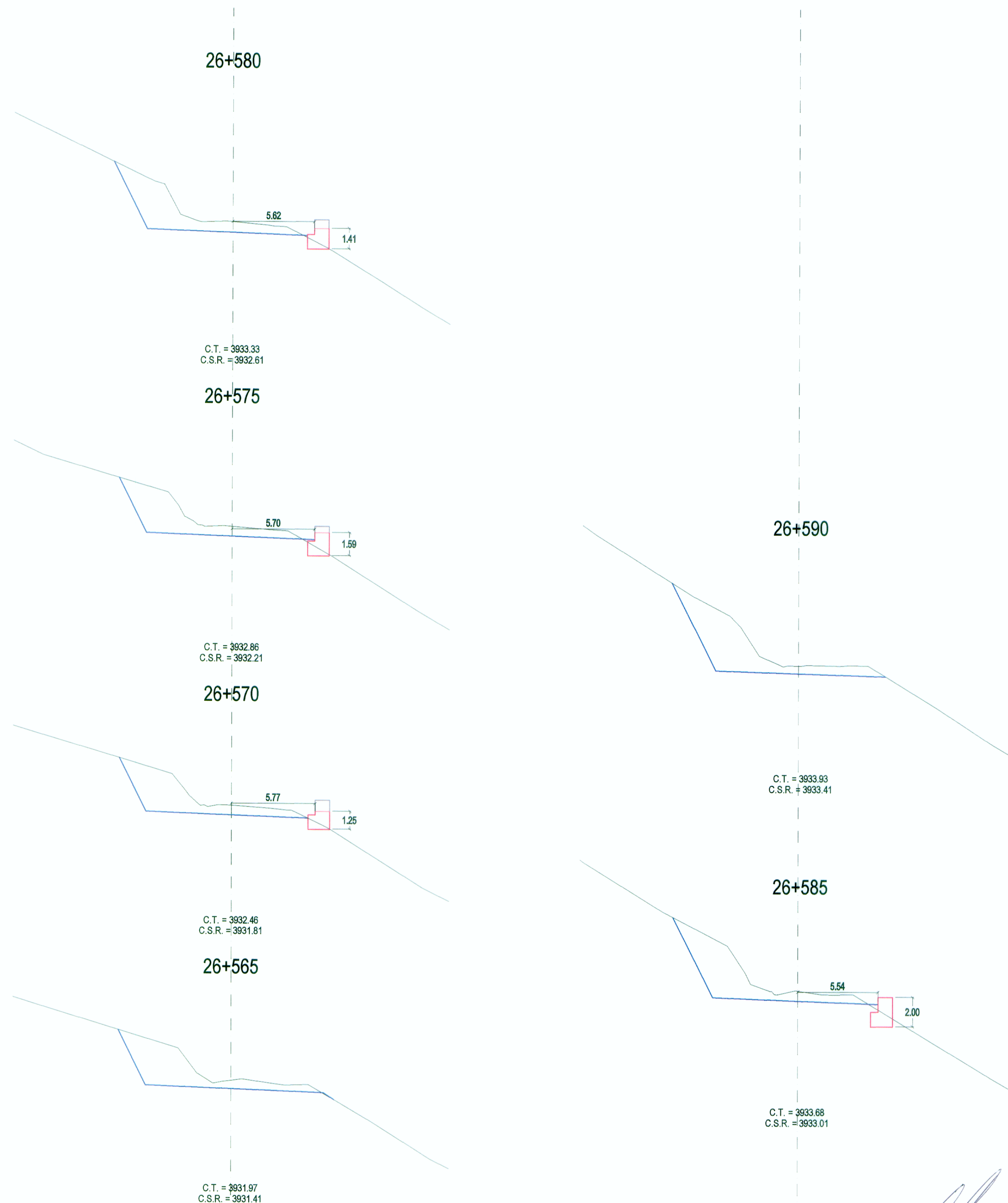
SECCIONES TRANSVERSALES
