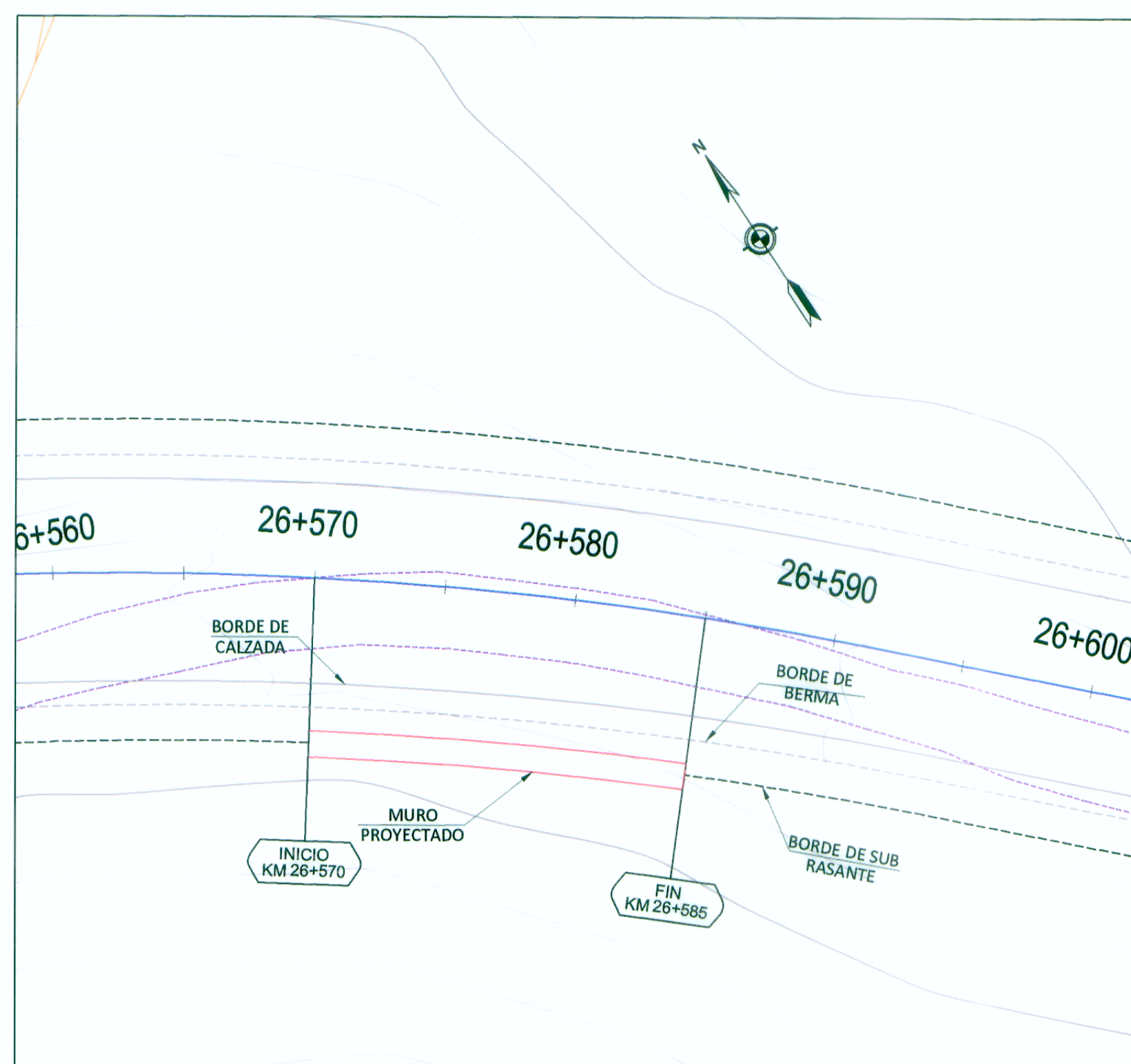
PLANTA
