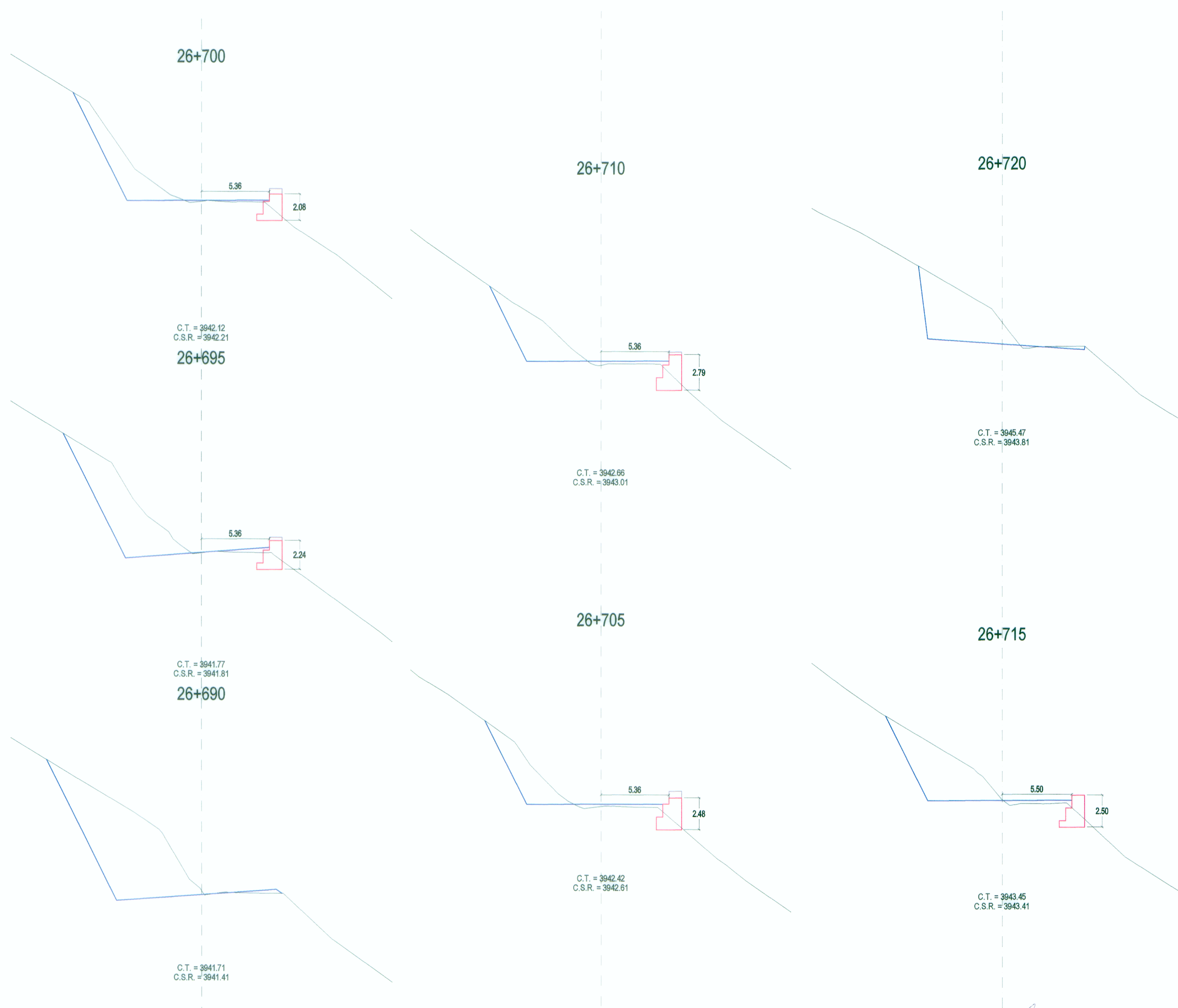
SECCIONES TRANSVERSALES
