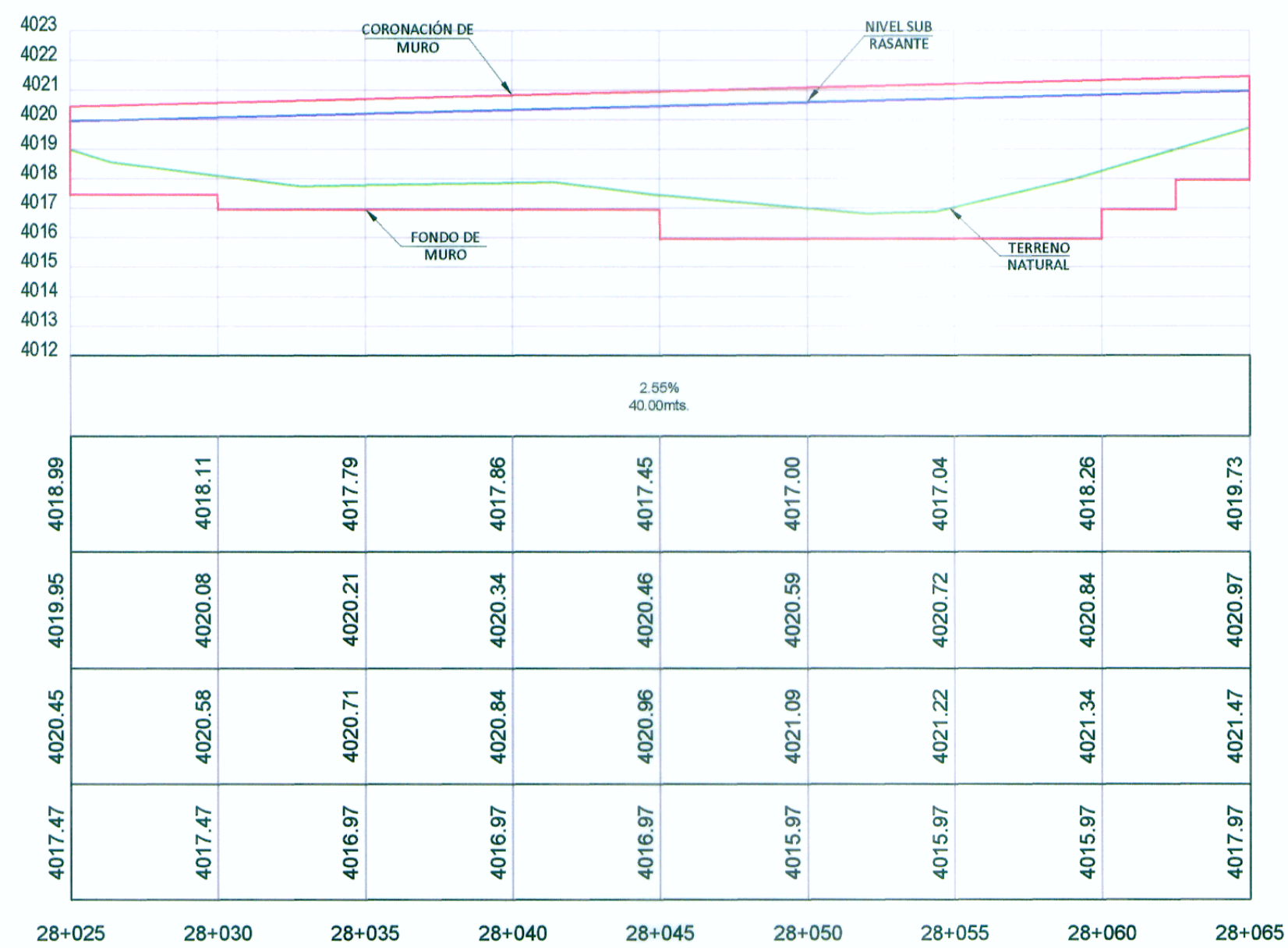
PERFIL LONGITUDINAL
