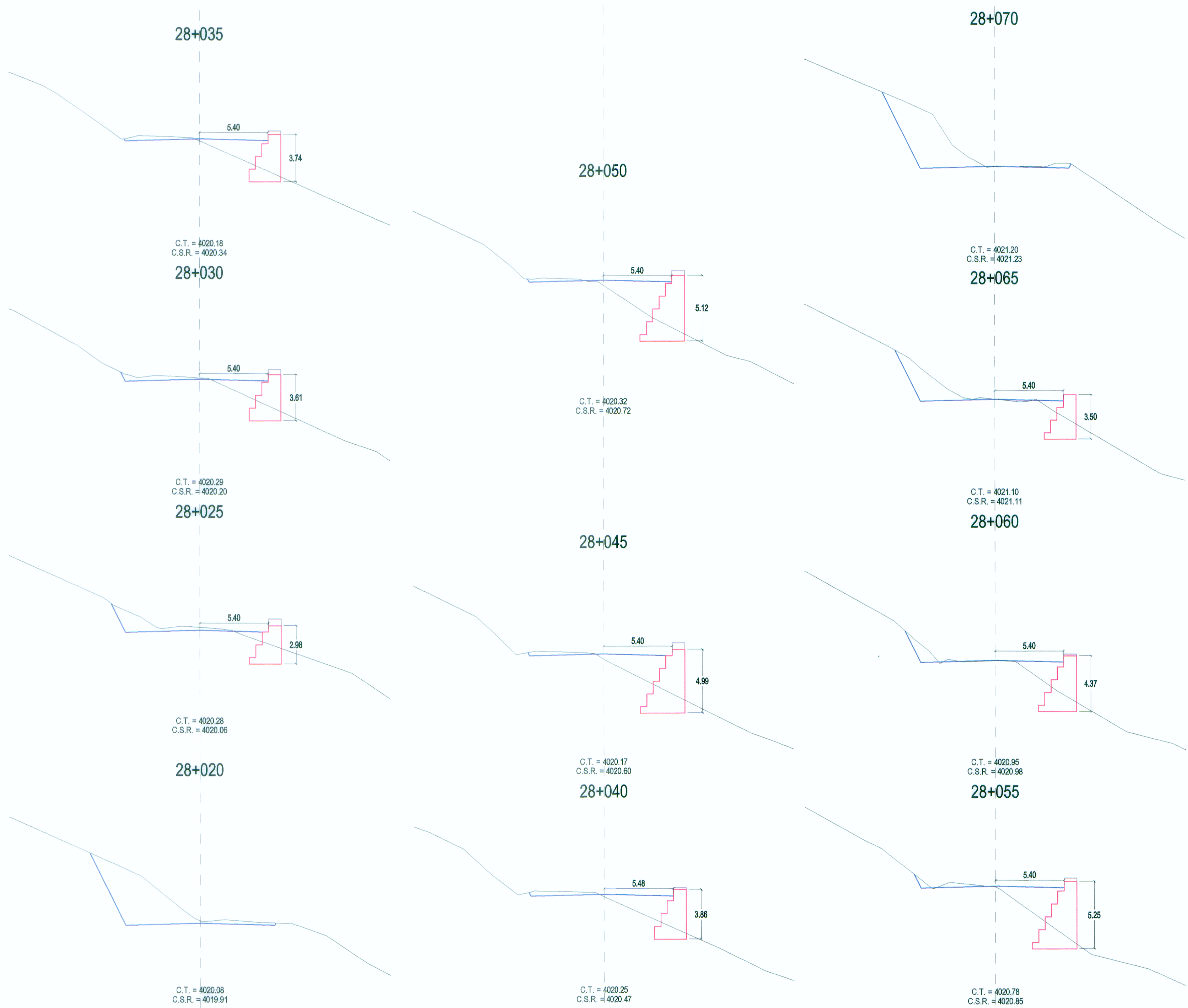
SECCIONES TRANSVERSALES
