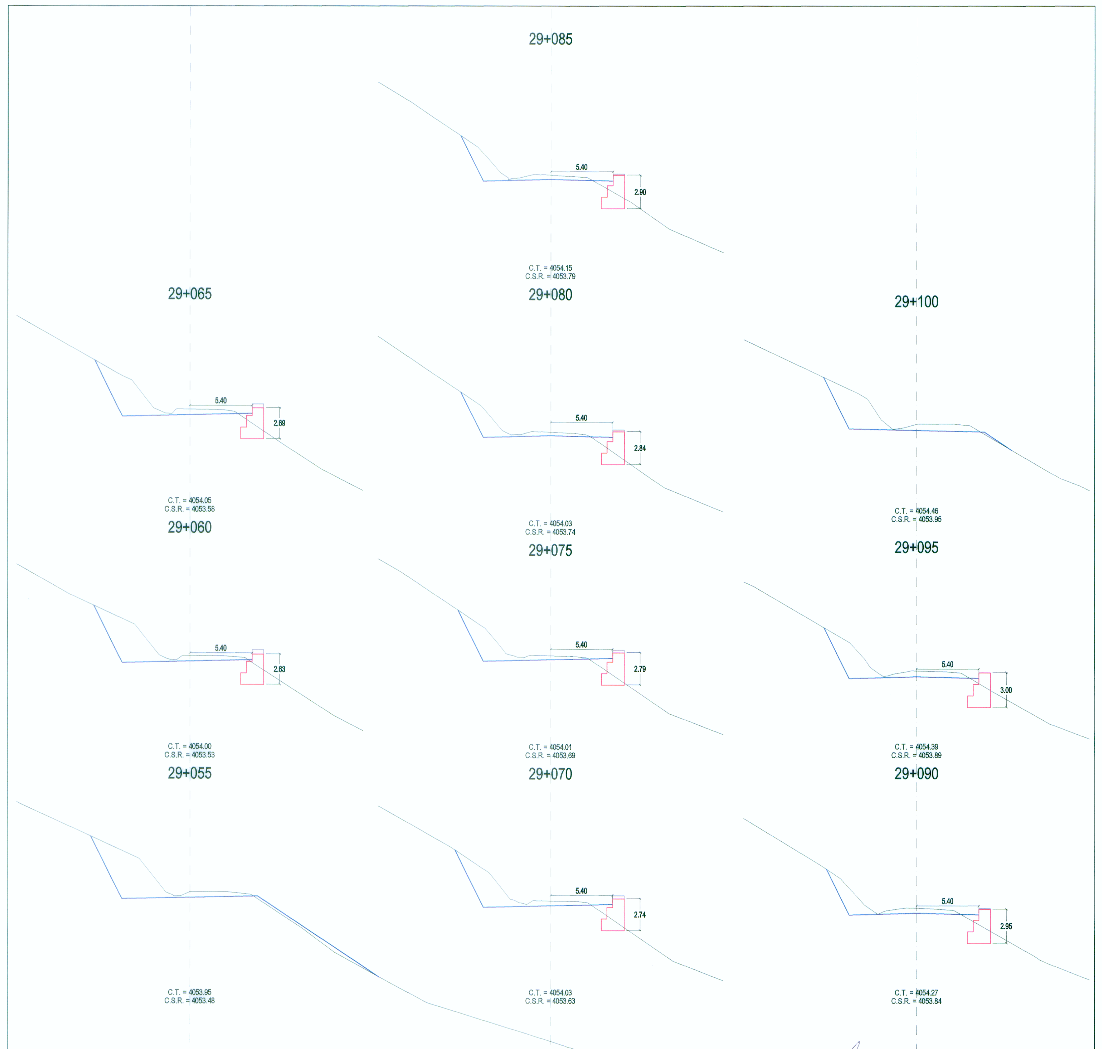
SECCIONES TRANSVERSALES
