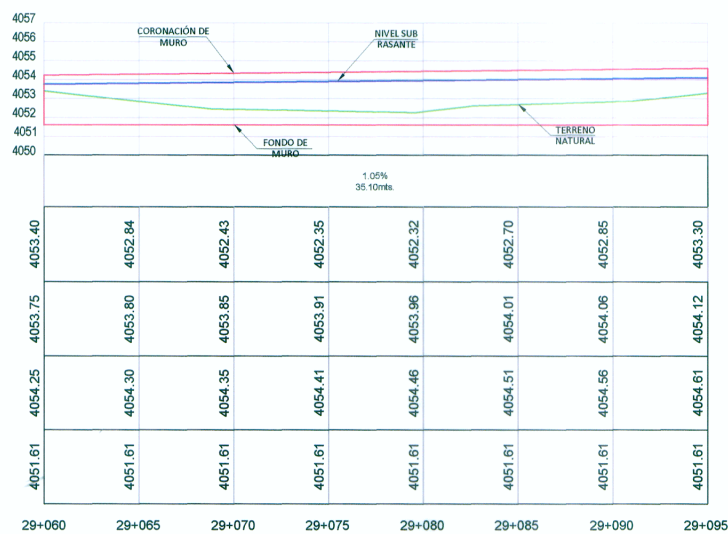
PERFIL LONGITUDINAL
