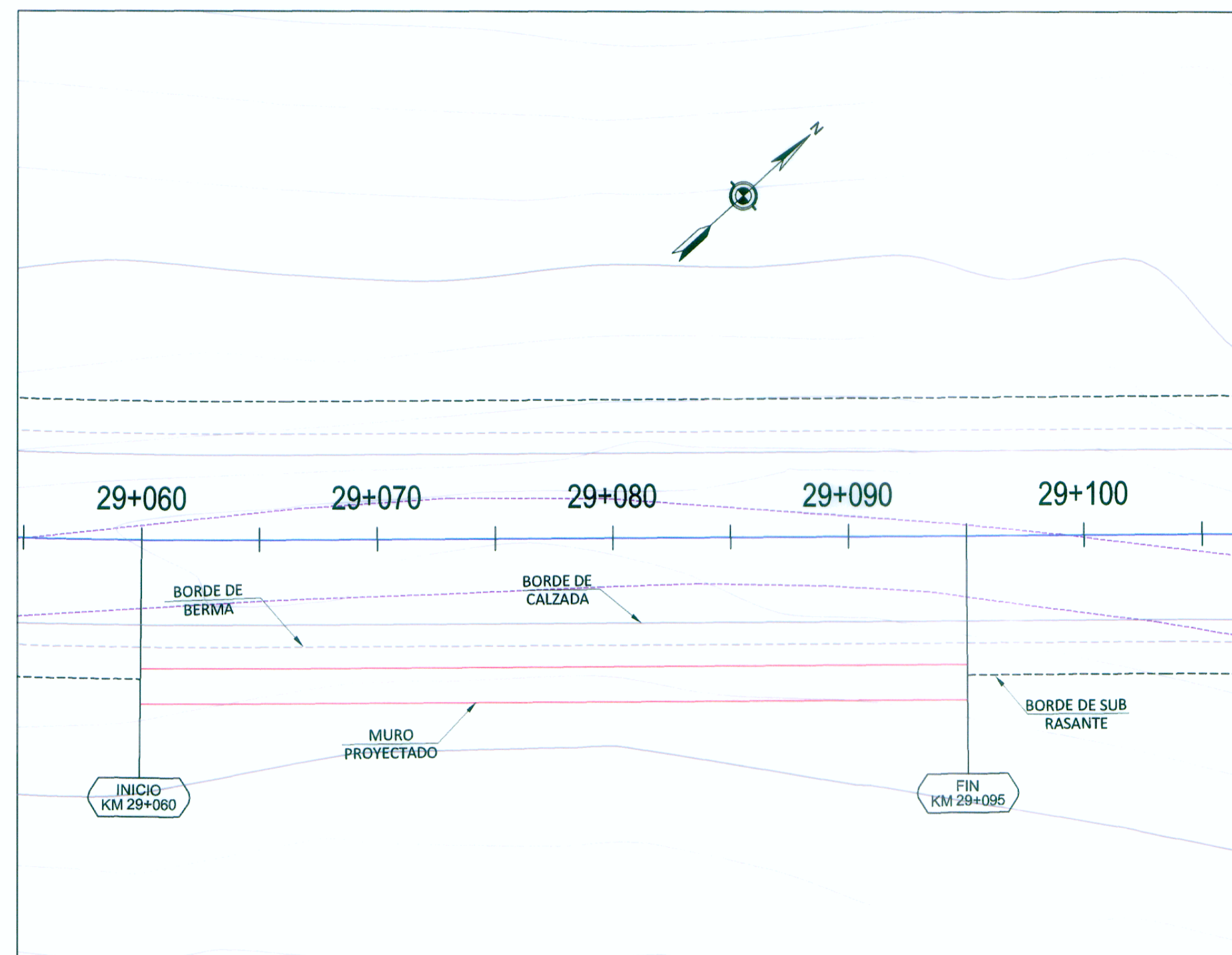
PLANTA
