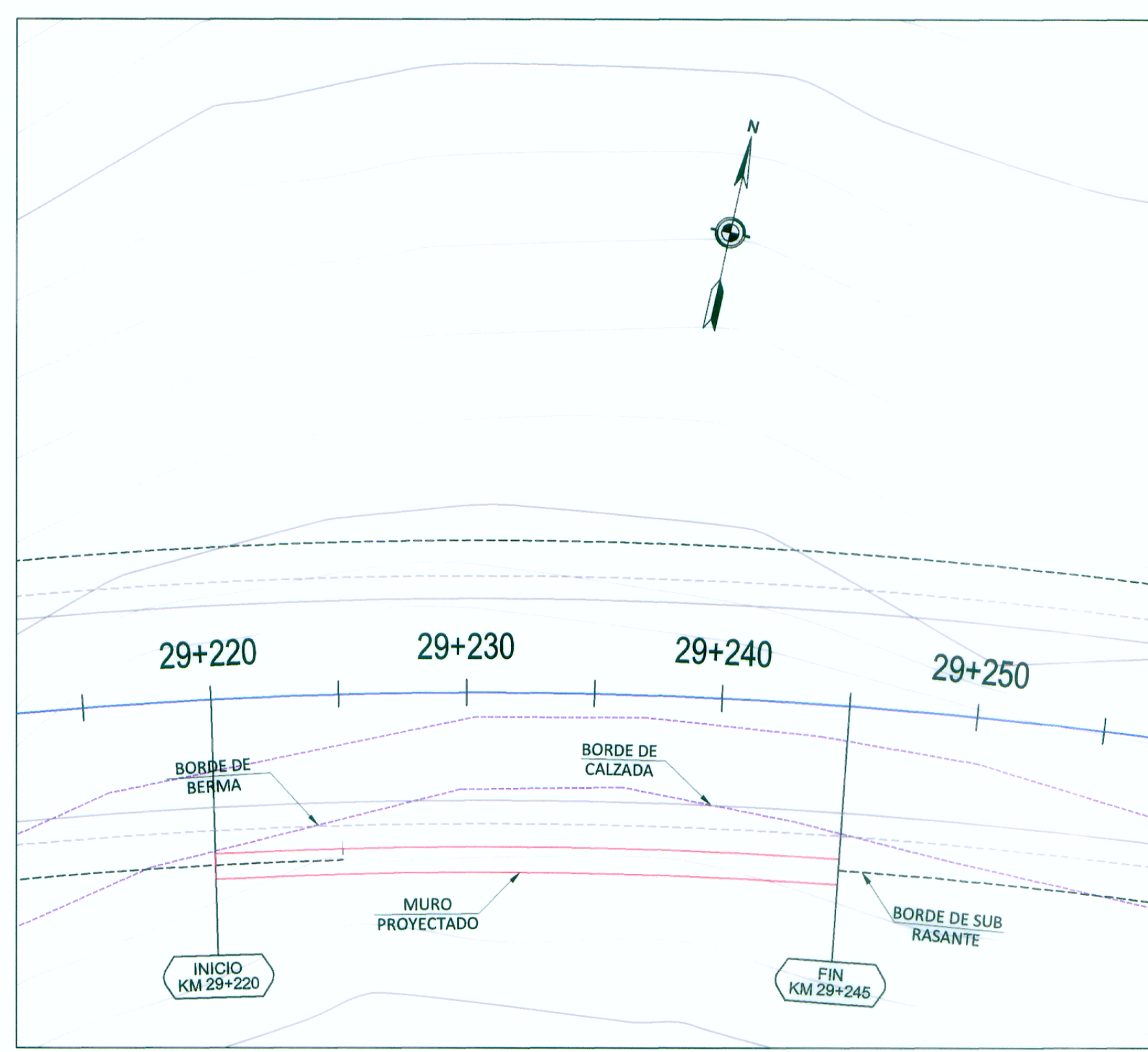
PLANTA
