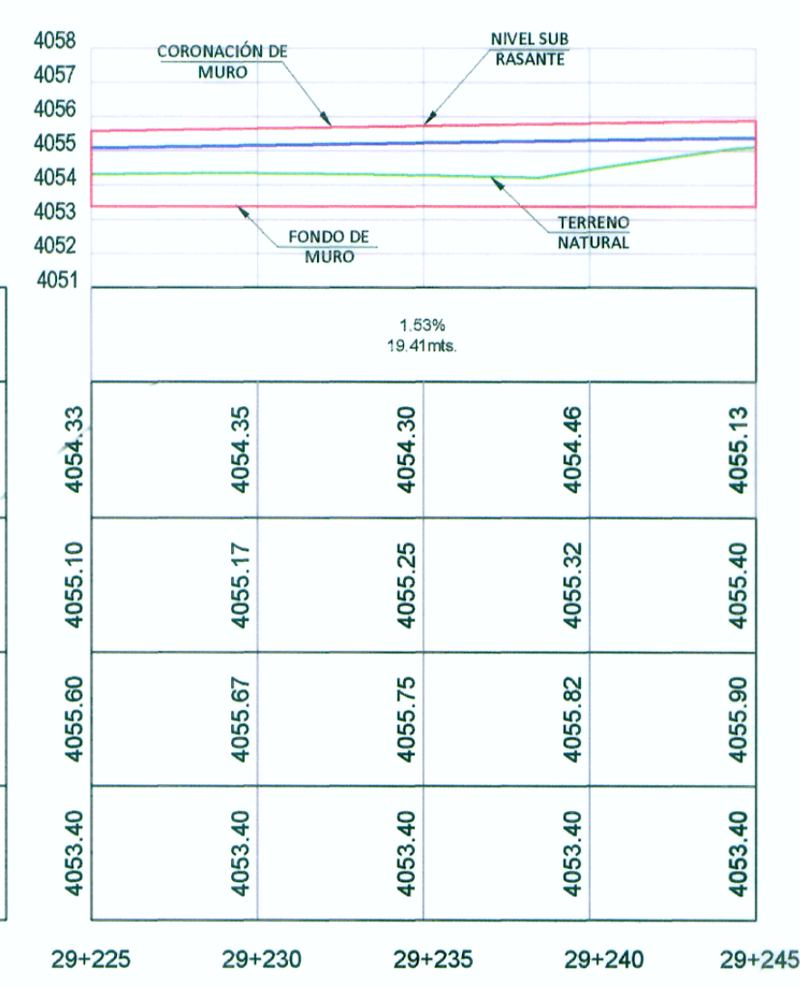
PERFIL LONGITUDINAL
