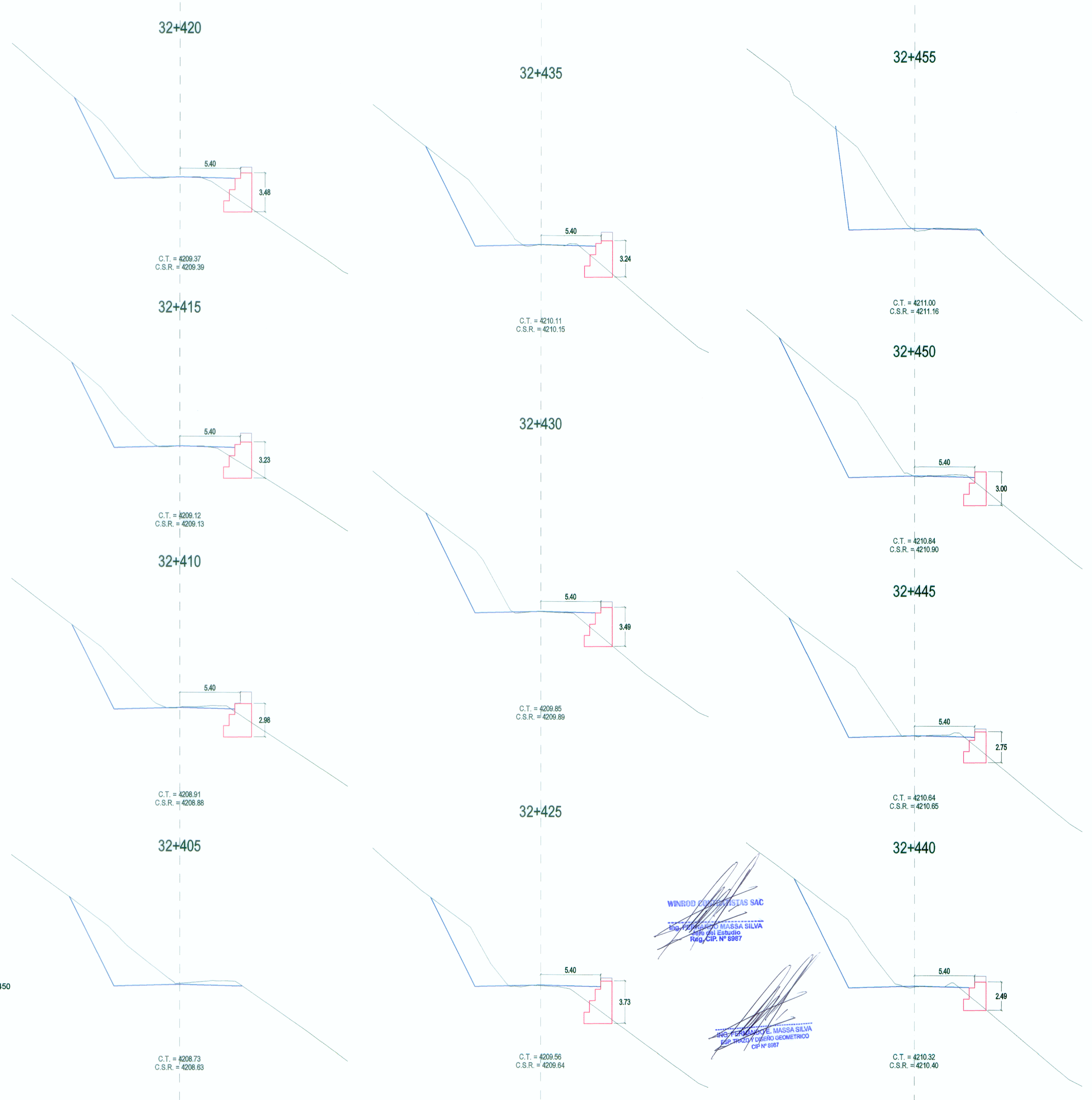
SECCIONES TRANSVERSALES
