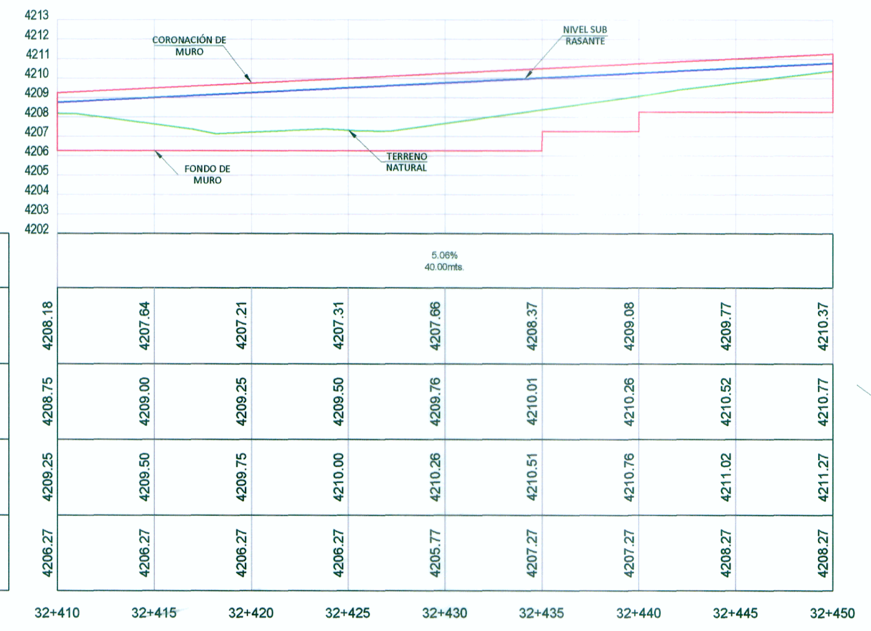
PERFIL LONGITUDINAL
