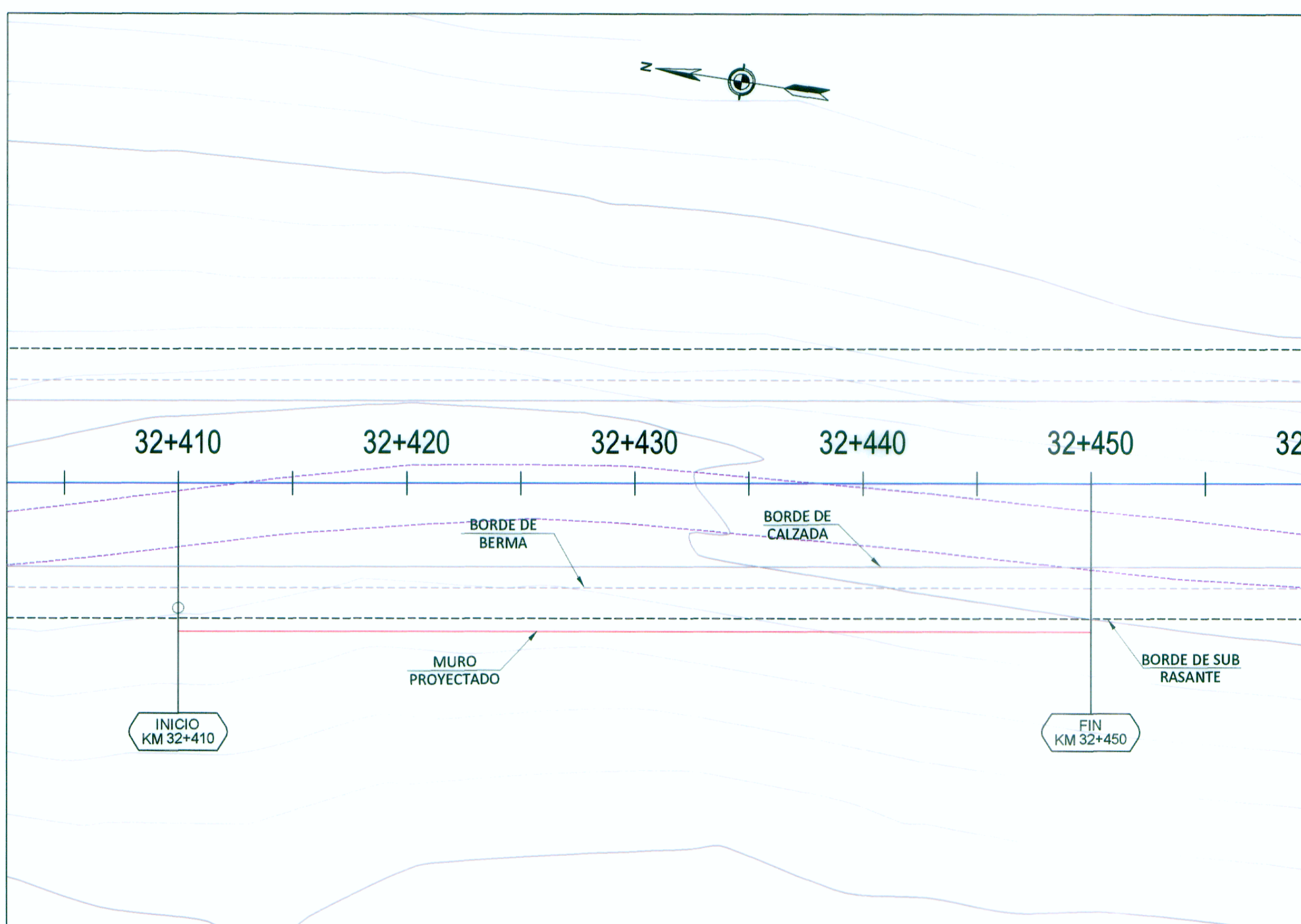
PLANTA
