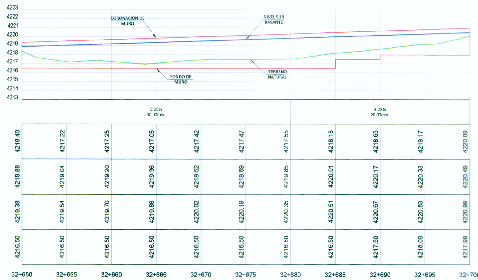
PERFIL LONGITUDINAL
