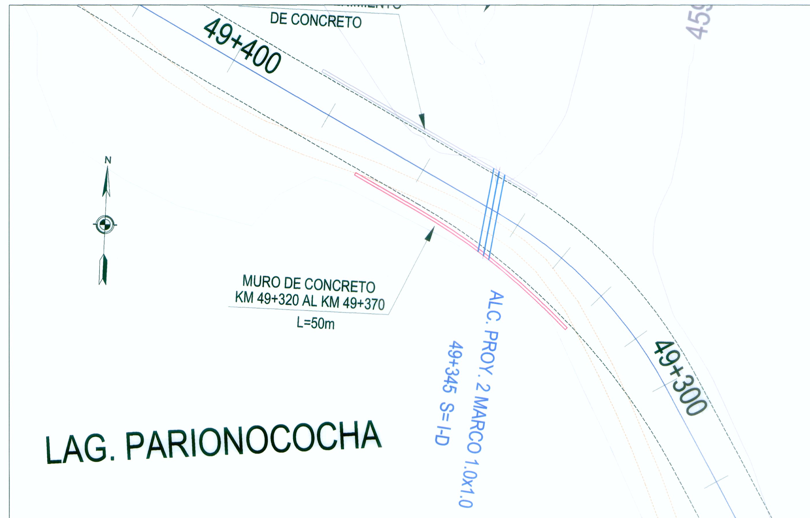
PLANTA
