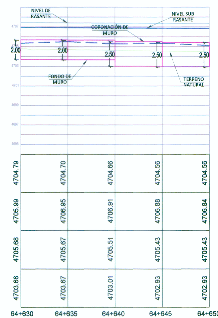
Muro Gavión 64+630 - 64+650
