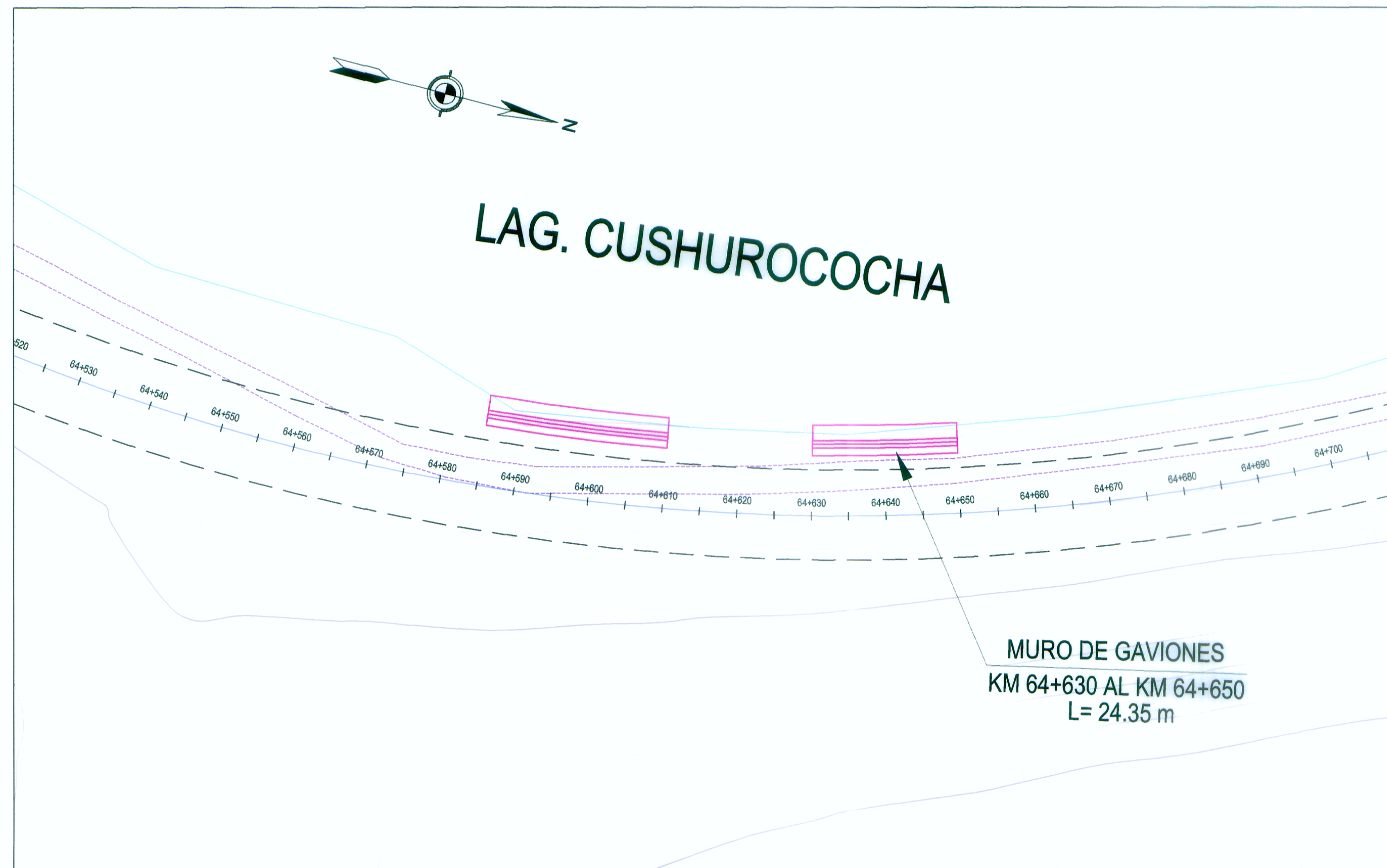
PLANTA
