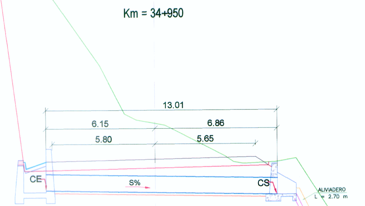
TMC Ø36" PROYECTADA Protección L=2.70 m
