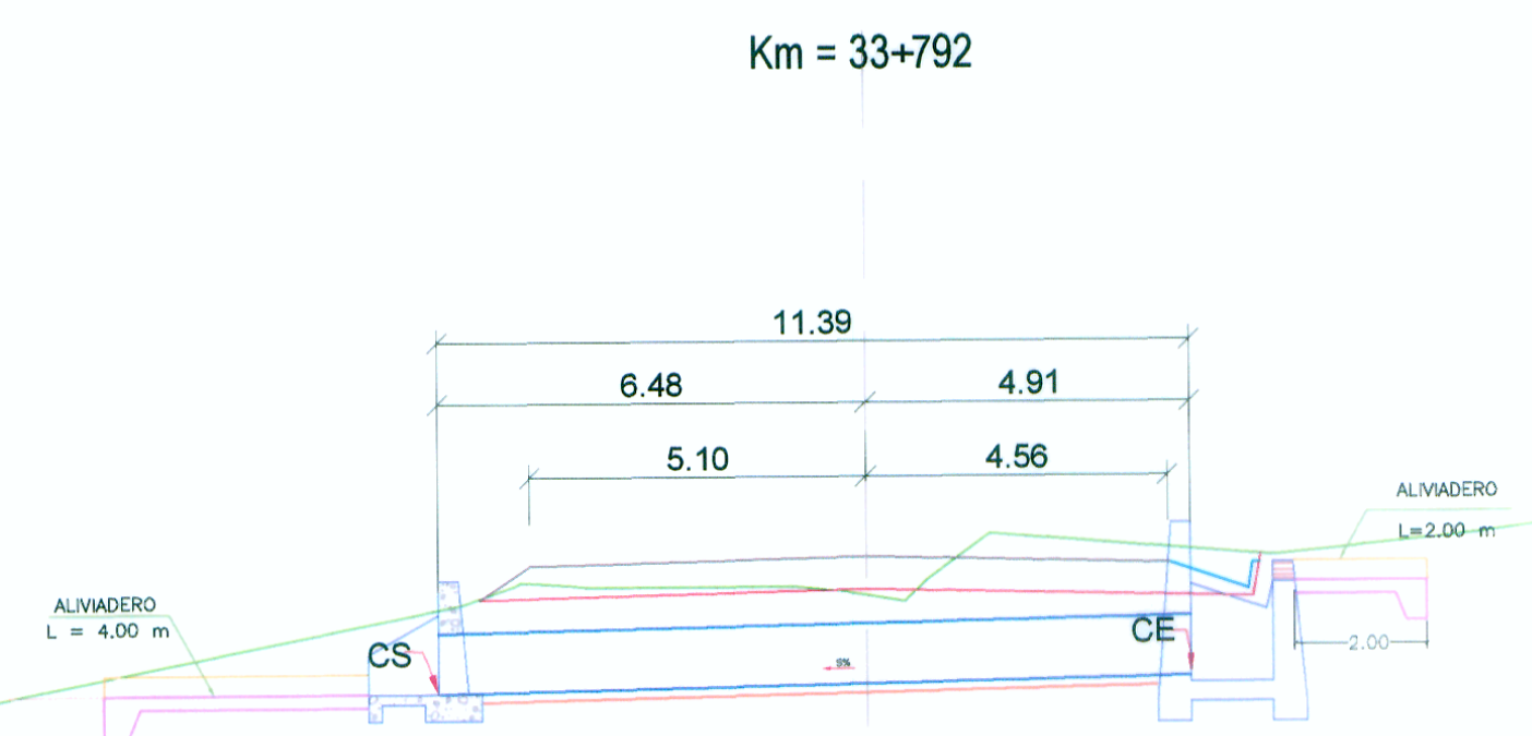
TMC Ø36" PROYECTADA Protección L=4.0 m Protección L=2.0 m
