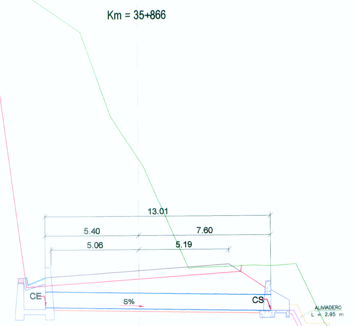
TMC Ø36" PROYECTADA Protección L = 2.95 m
