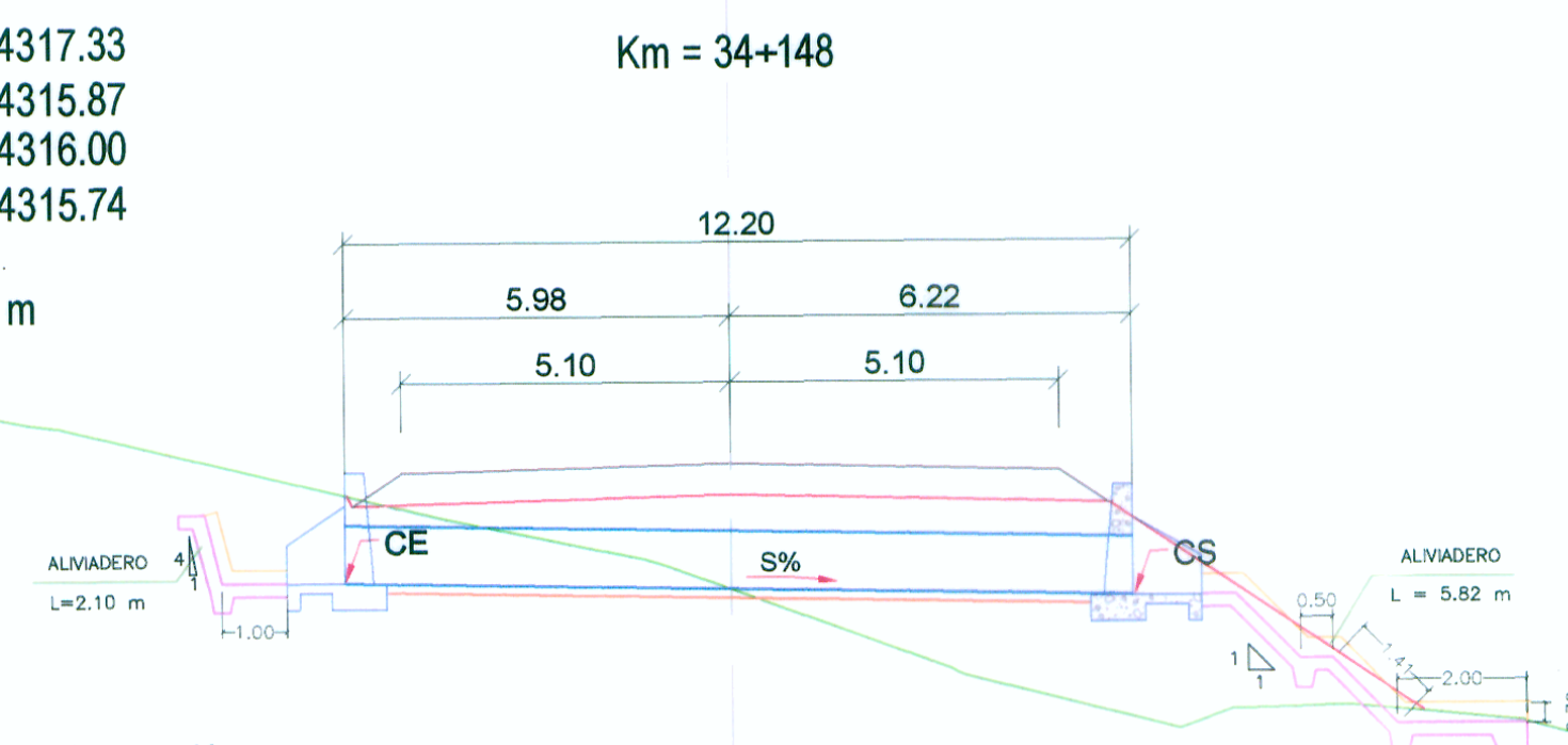
TMC Ø36" PROYECTADA Protección L=2.10 m Protección L=5.82 m
