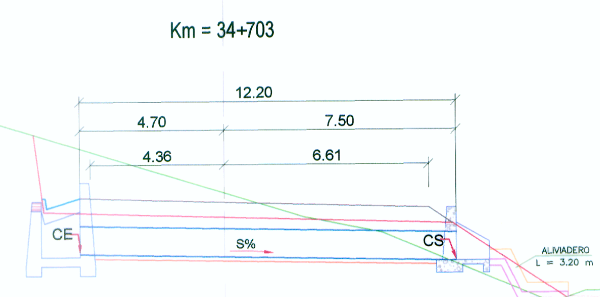
TMC Ø36" PROYECTADA Protección L=3.2 m
