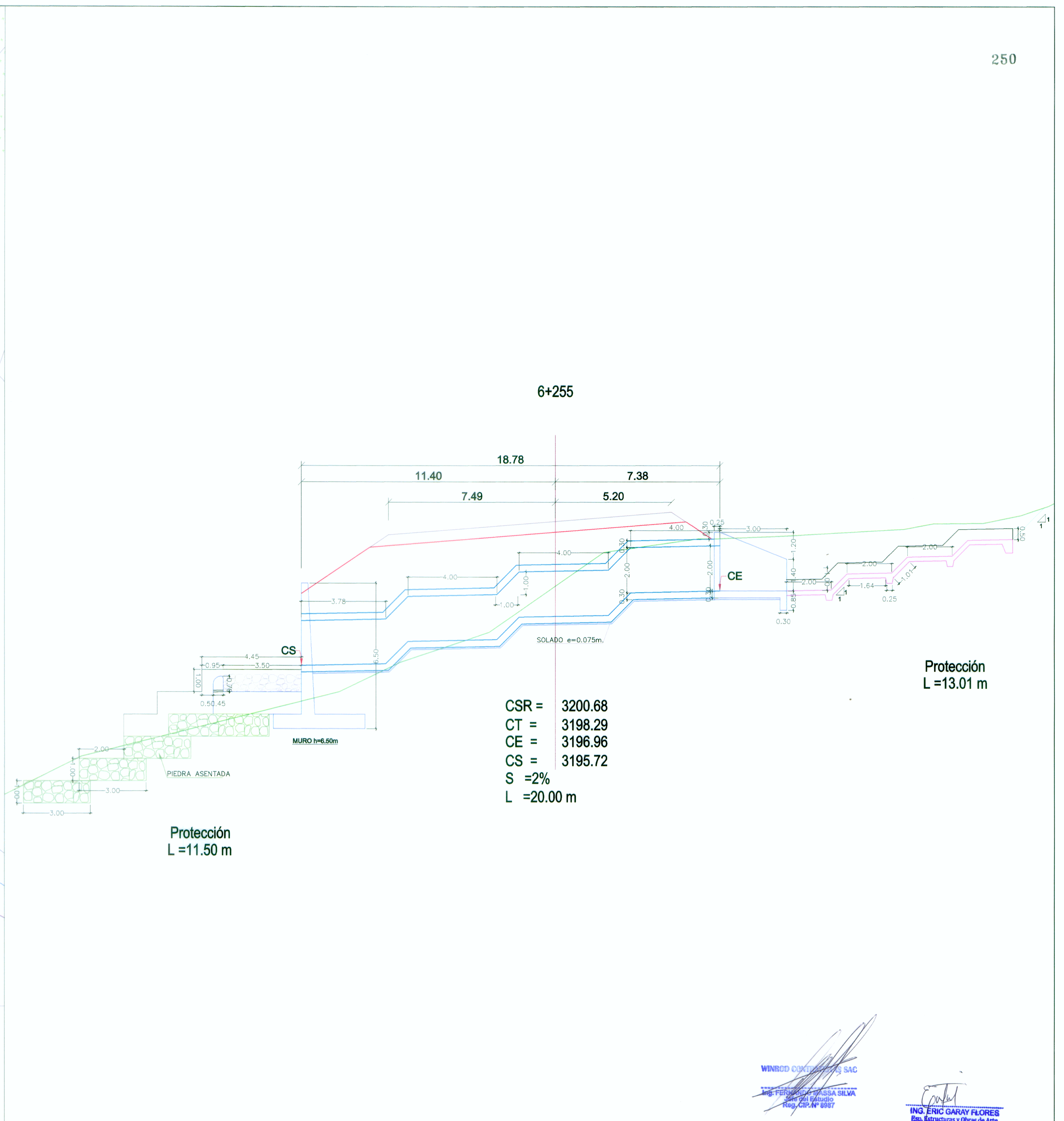
SECCIÓN TRANSVERSAL Esc: 1/100
