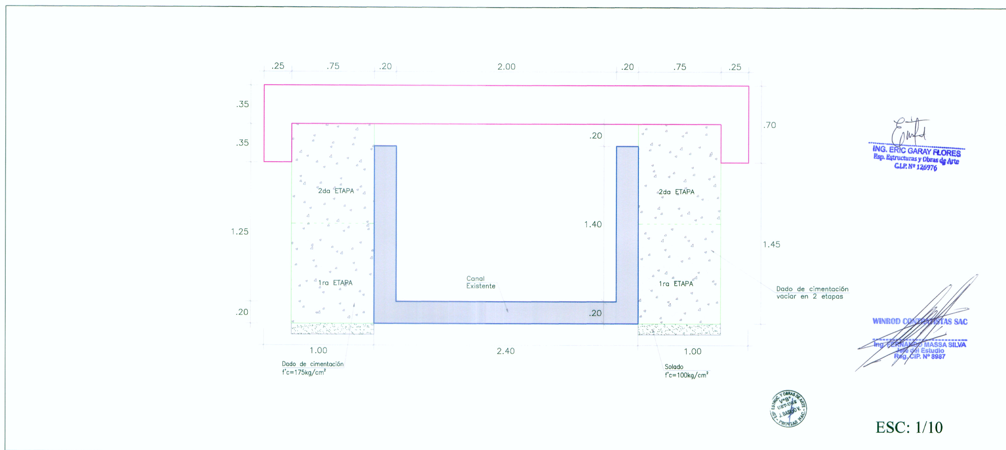
SECCIÓN DE LOSA SOBRE CANAL EXISTENTE
