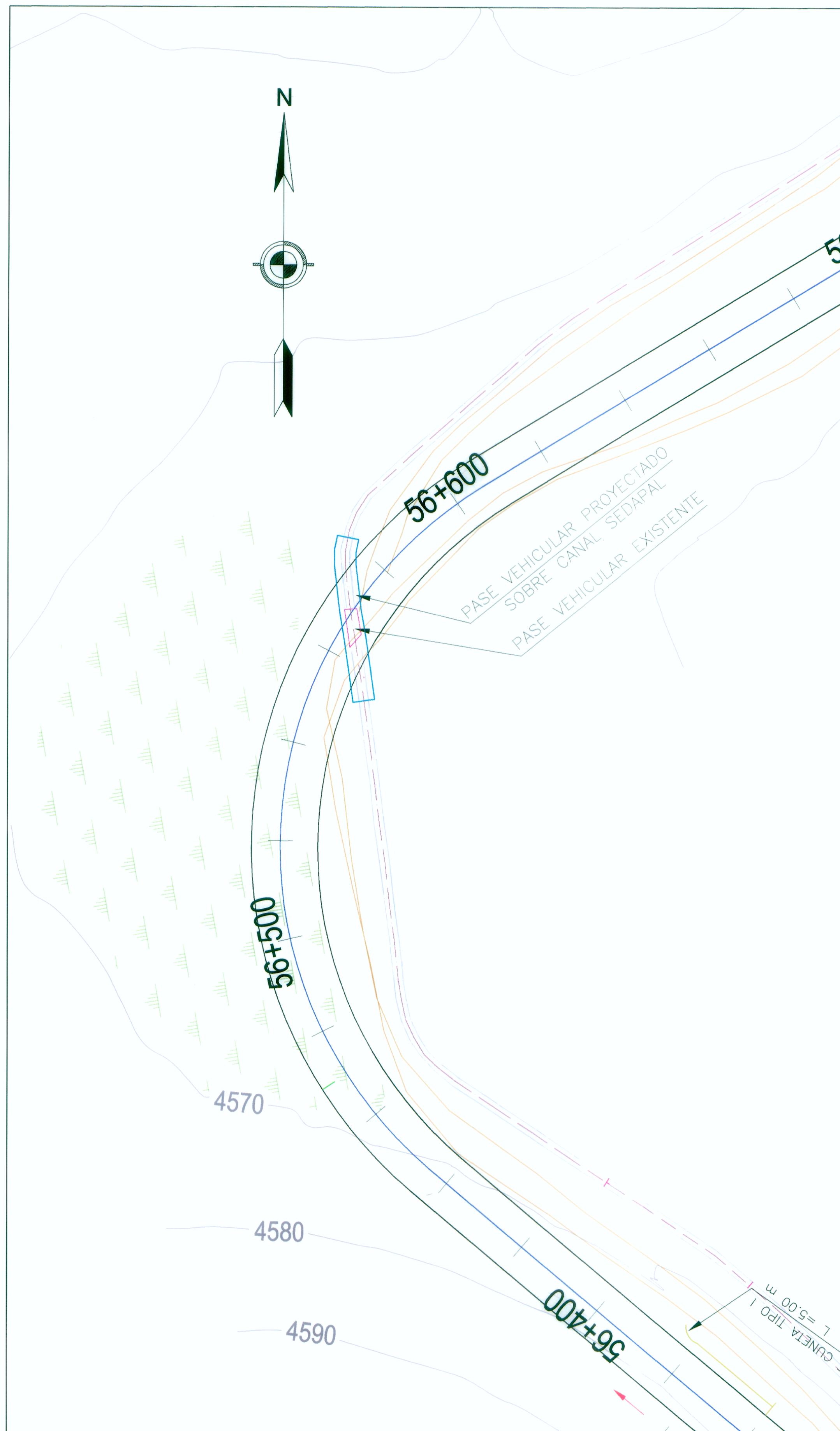
UBICACIÓN ESC: 1/300
