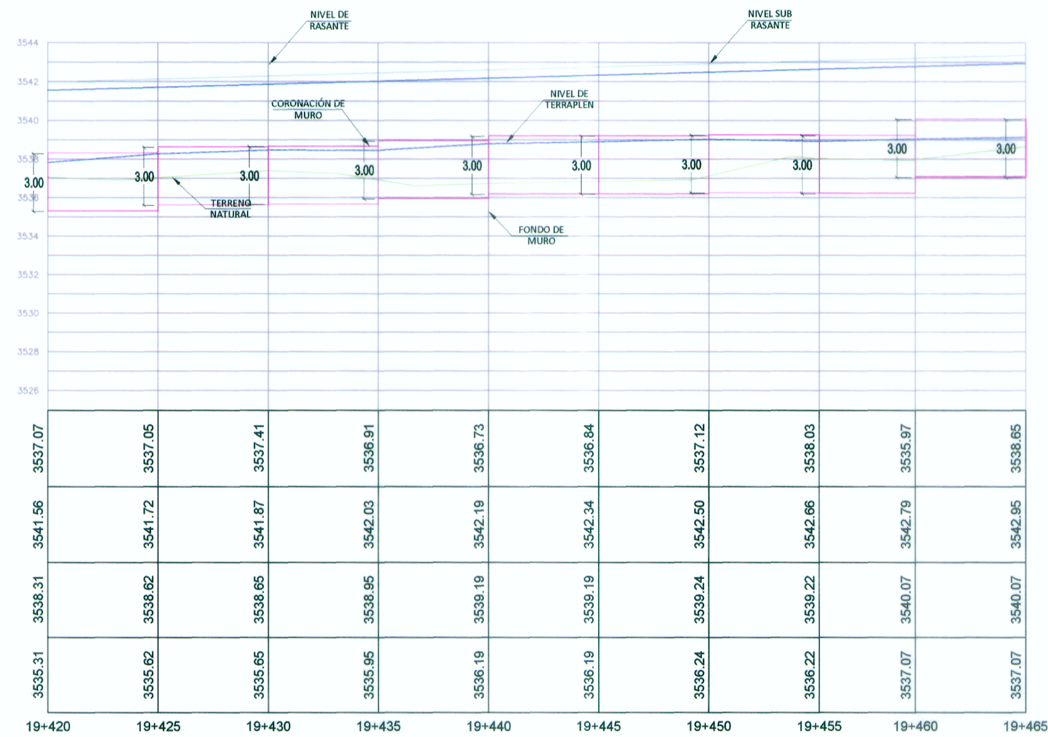
Muro Gavión 19+420 - 19+465
