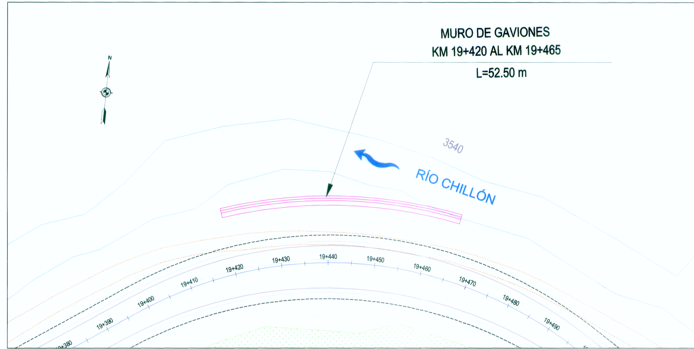
PLANTA
