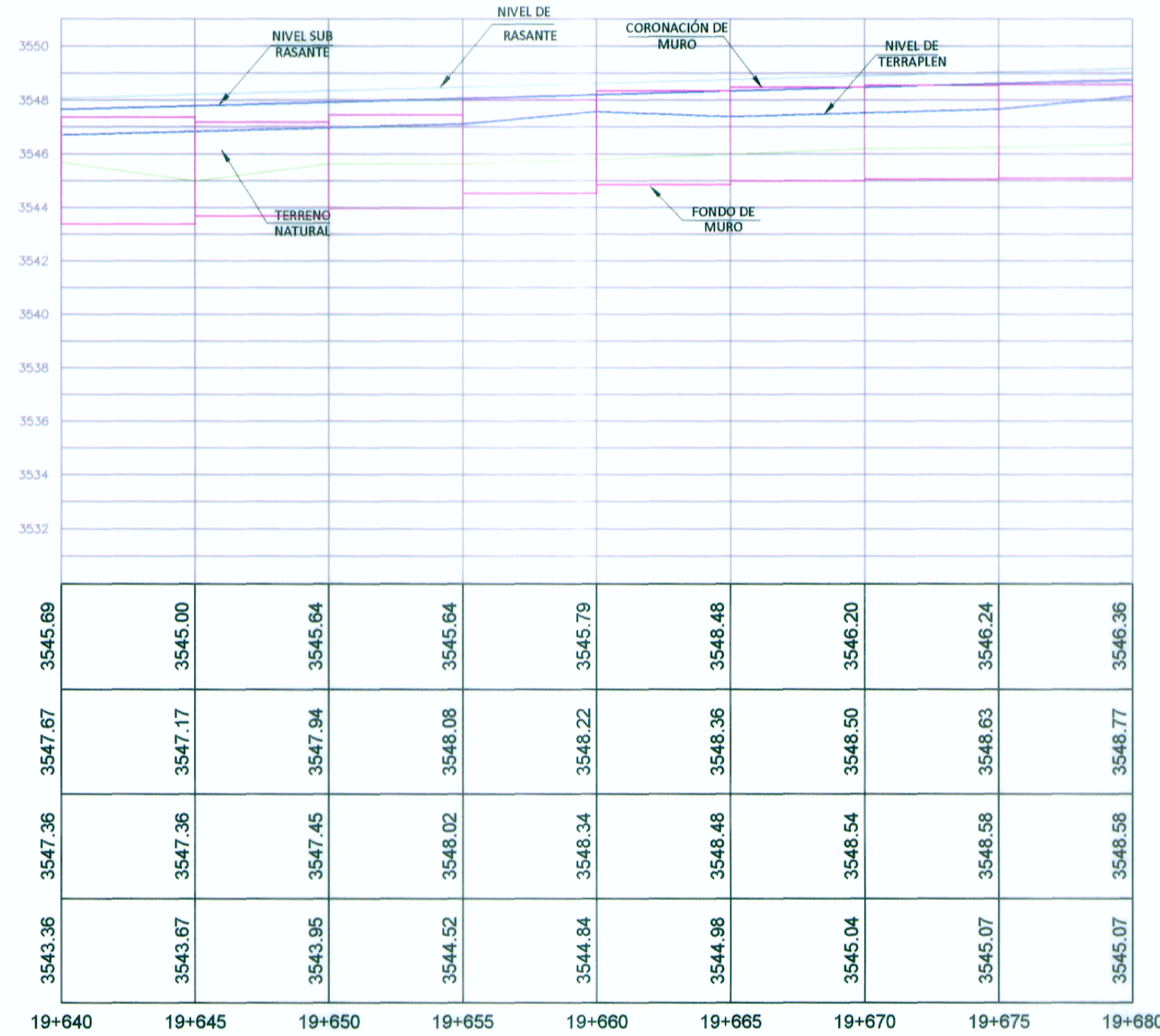
Muro Gavión 19+640 - 19+680
