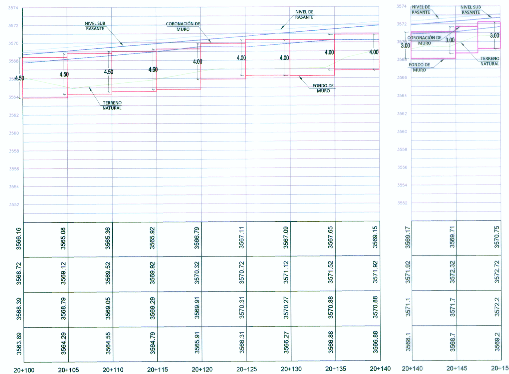
Muro Concreto y Muro Gavión 20+100 - 20+150
