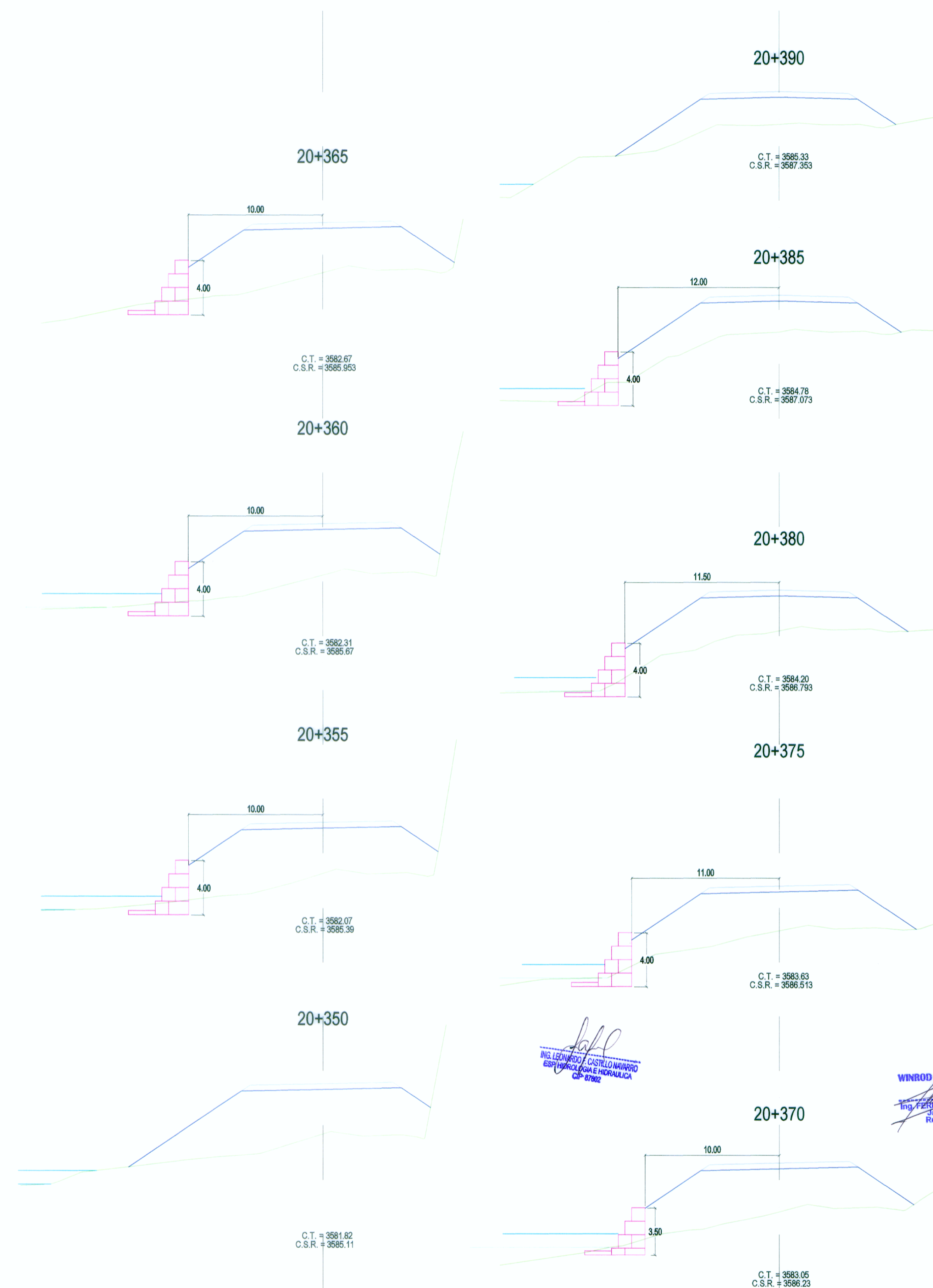
SECCIONES TRANSVERSALES Esc. 1/200
