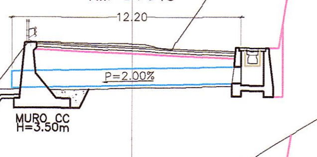
ALCANTARILLA TIPO TMC Ø36" REEMPLAZAR KM 3+640
