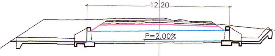
ALCANTARILLA TIPO TMC 36" PROYECTAR KM 10+345
