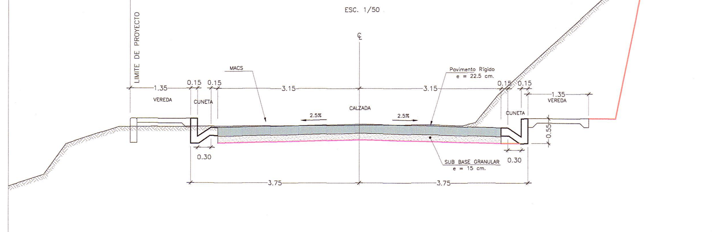
SECCION TIPO ZONA URBANA (Por empalme a proyecto de la Municipalidad Provincial de Huancavelica Km. 0+000 - Km. 1+550) HUANCAVELICA Km 1+550 - Km 1+700 ESC. 1/50
