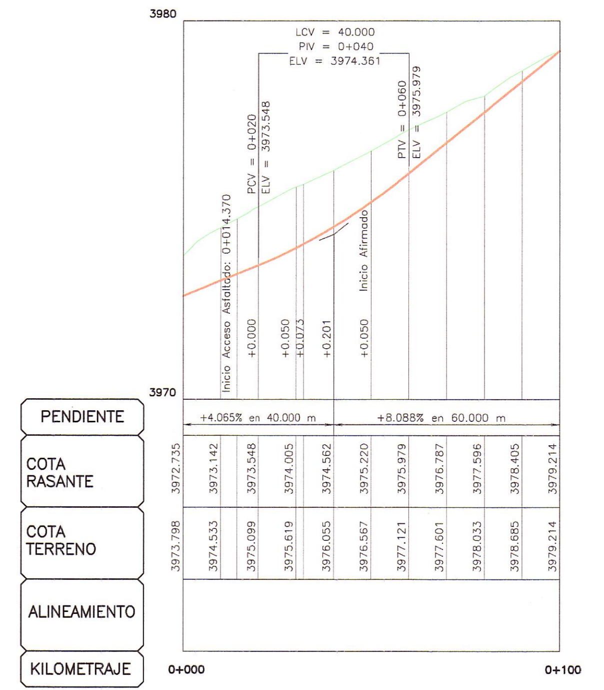
PERFIL 1:1000
