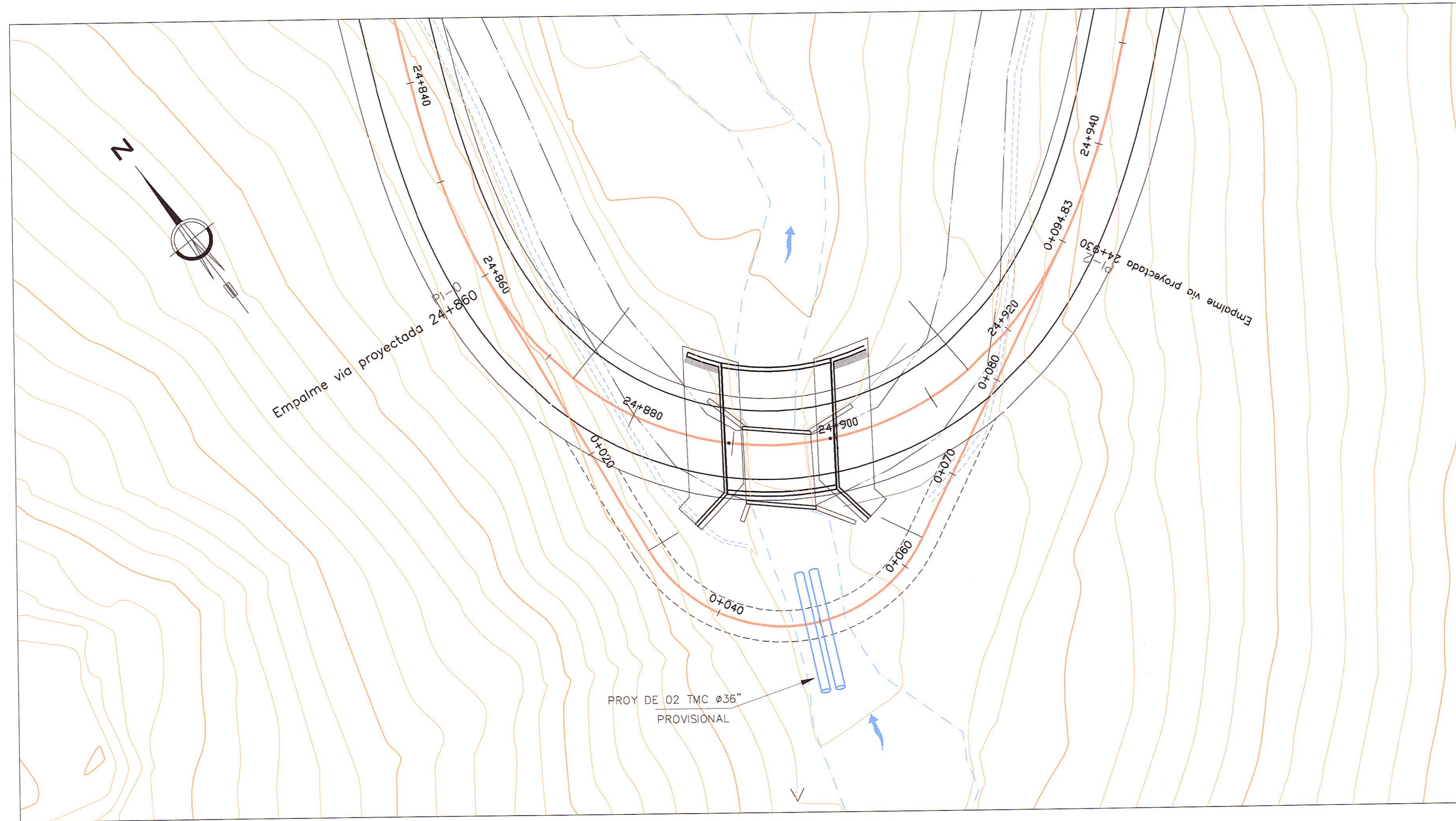
PLANTA 1:300
