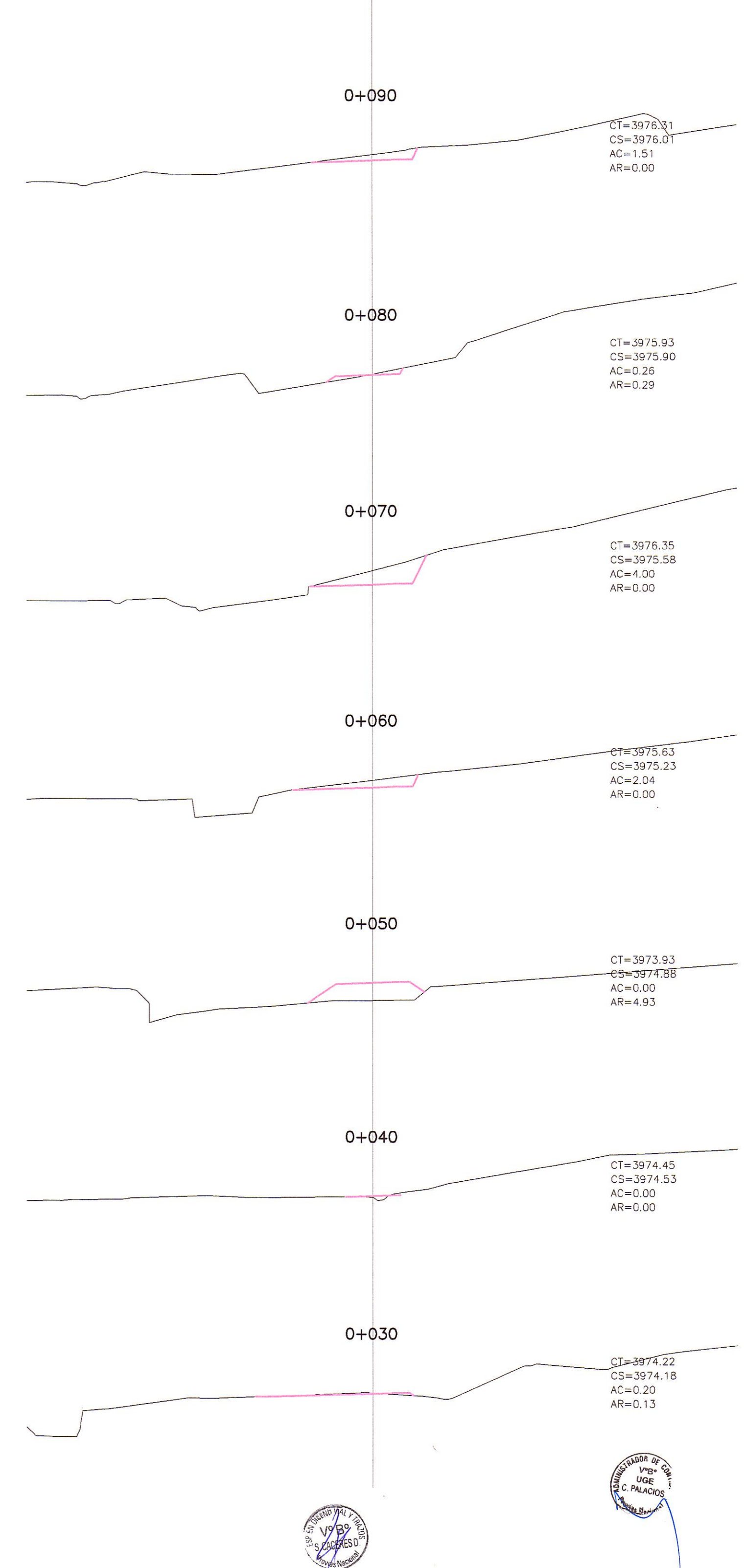
SECCIONES 1:200
