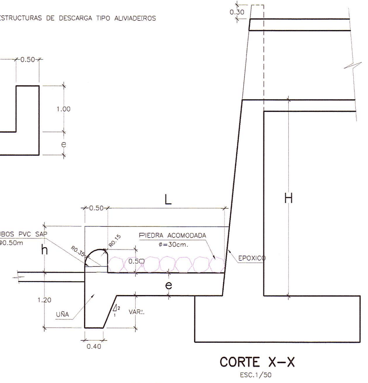
DISIPADOR DE ENERGIA DE ALCANTARILLA MARCO DE 1.50X1.50 H>1.50m
