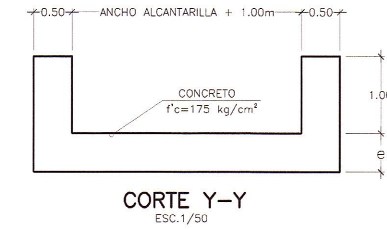
DISIPADOR DE ENERGIA DE ALCANTARILLA MARCO DE 1.50X1.50 H>1.50m
