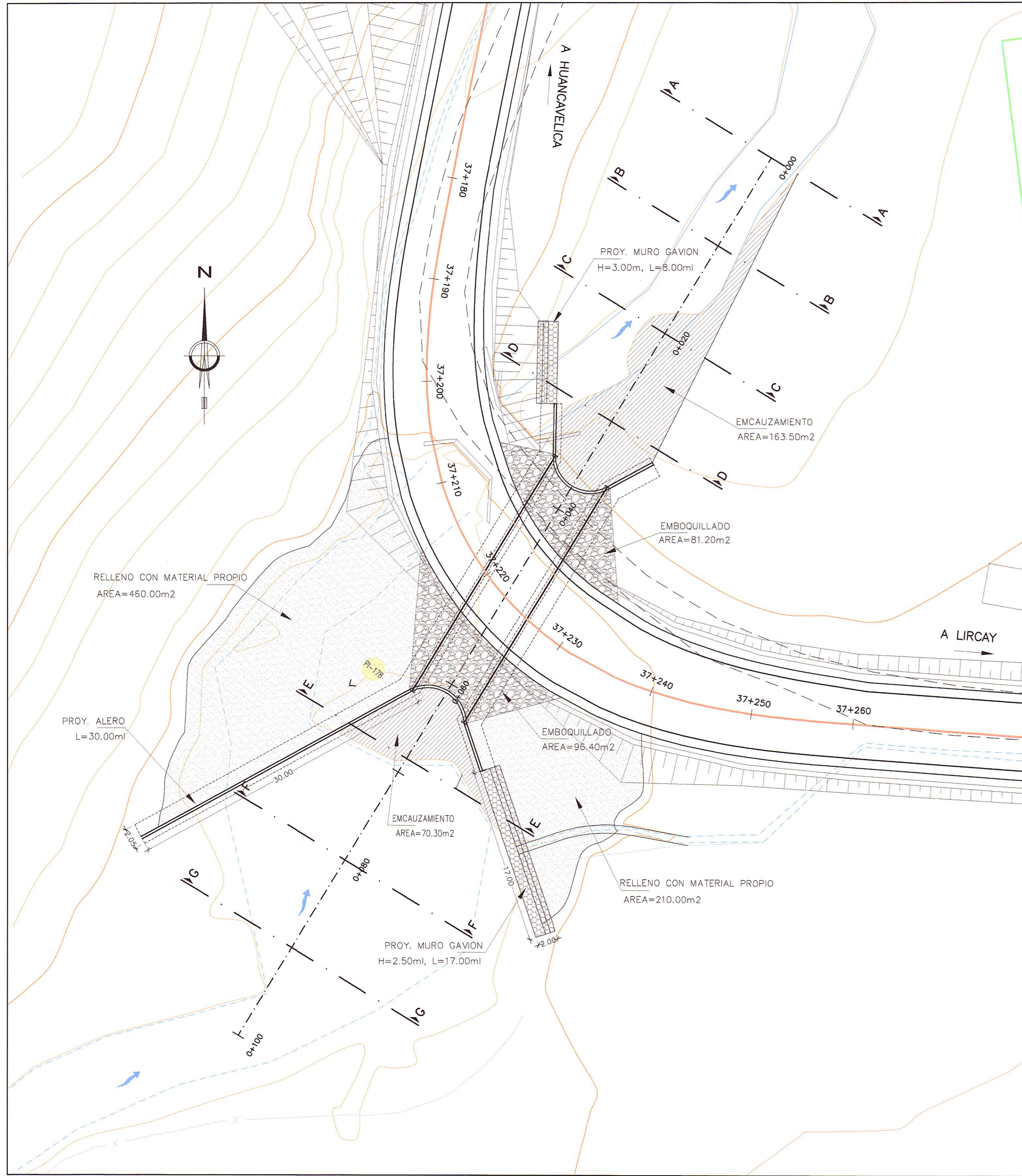
UBICACION Esc. 1/250
