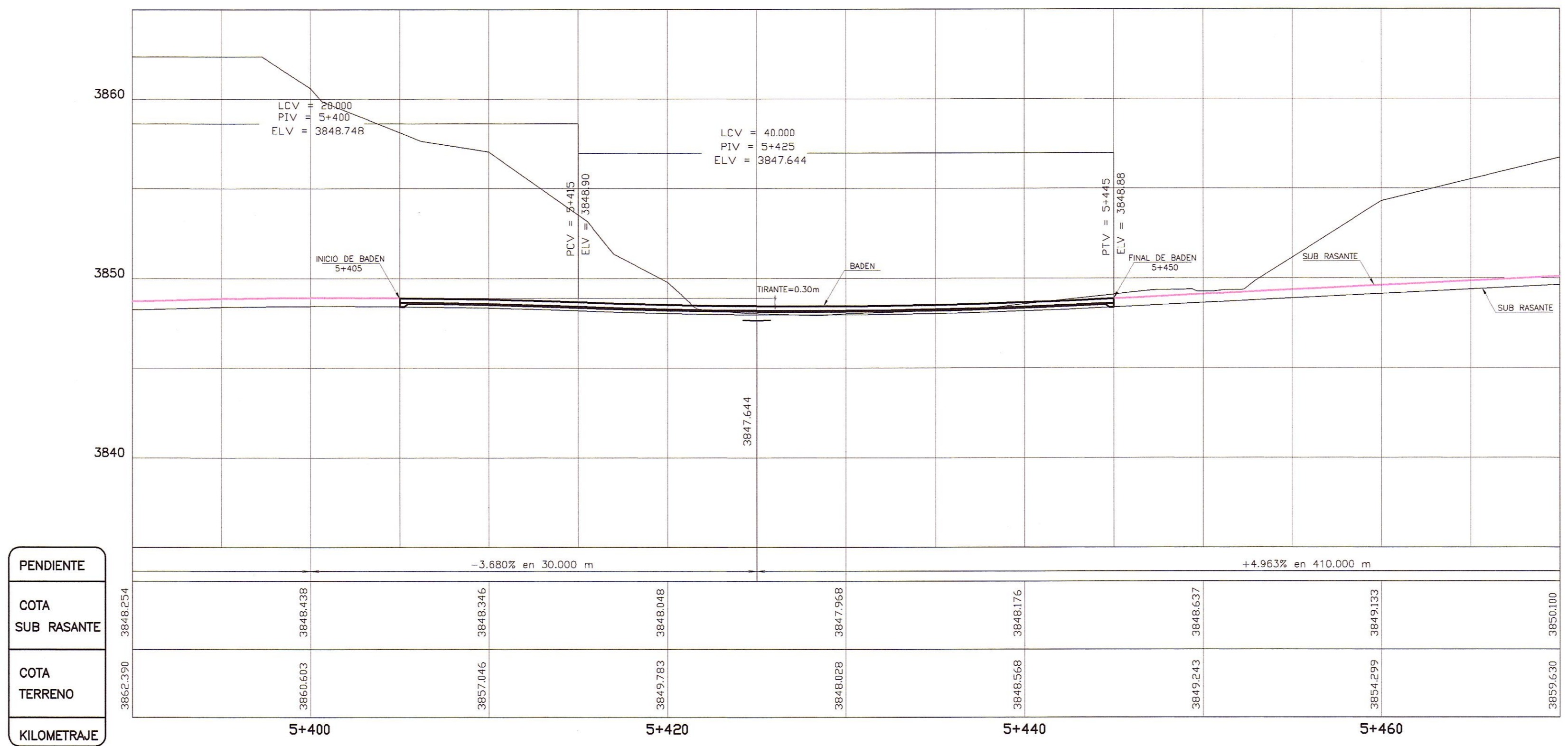
PERFIL LONGITUDINAL EJE DE LA CARRETERA ESC. 1/200
