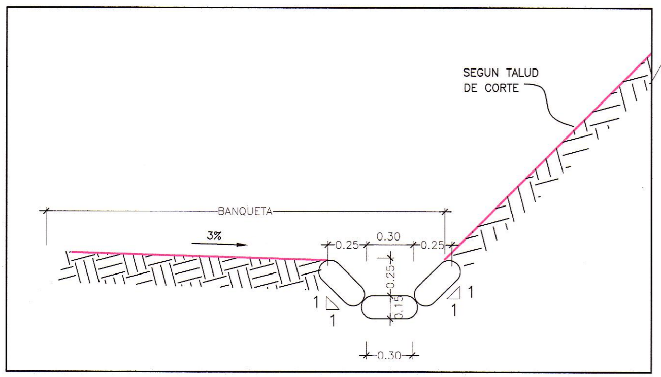
DETALLE DE CUNETA DE CORONACION SUELO CEMENTO ESC. 1/25
