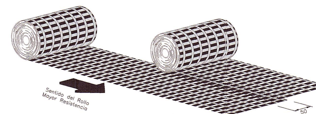
DETALLE DE SUPERPOSICIÓN DE GEOMALLA Sin Escala
