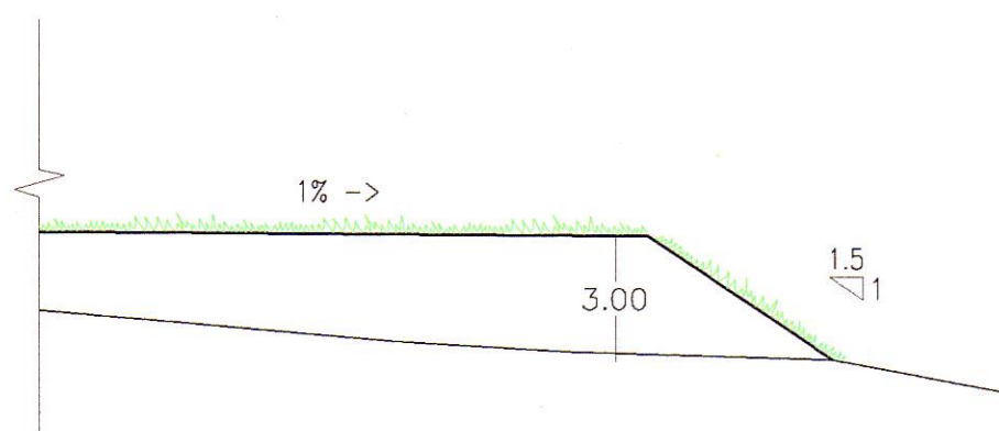
SECCION TIPICA DE BANQUETA 1:200
