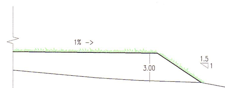
SECCION TIPICA DE BANQUETA 1:200
