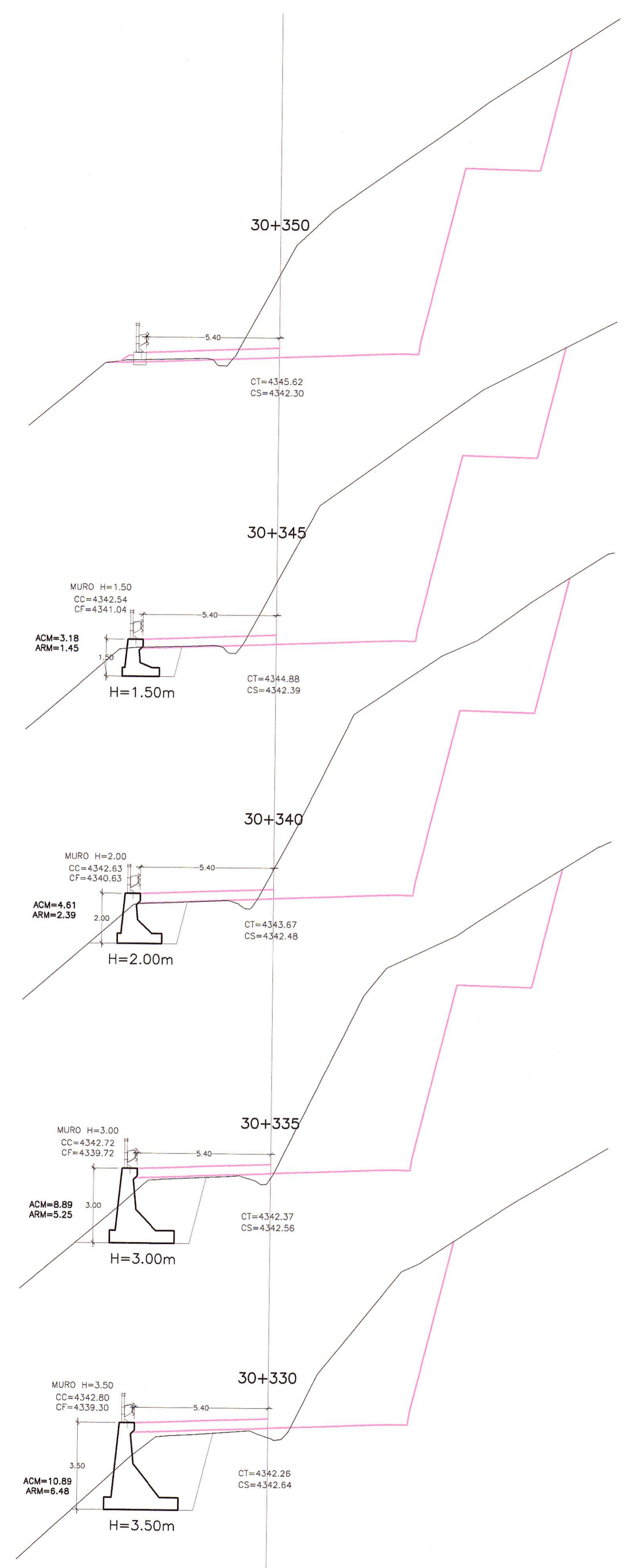
SECCIONES TRANSVERSALES ESC. 1: 1/125
