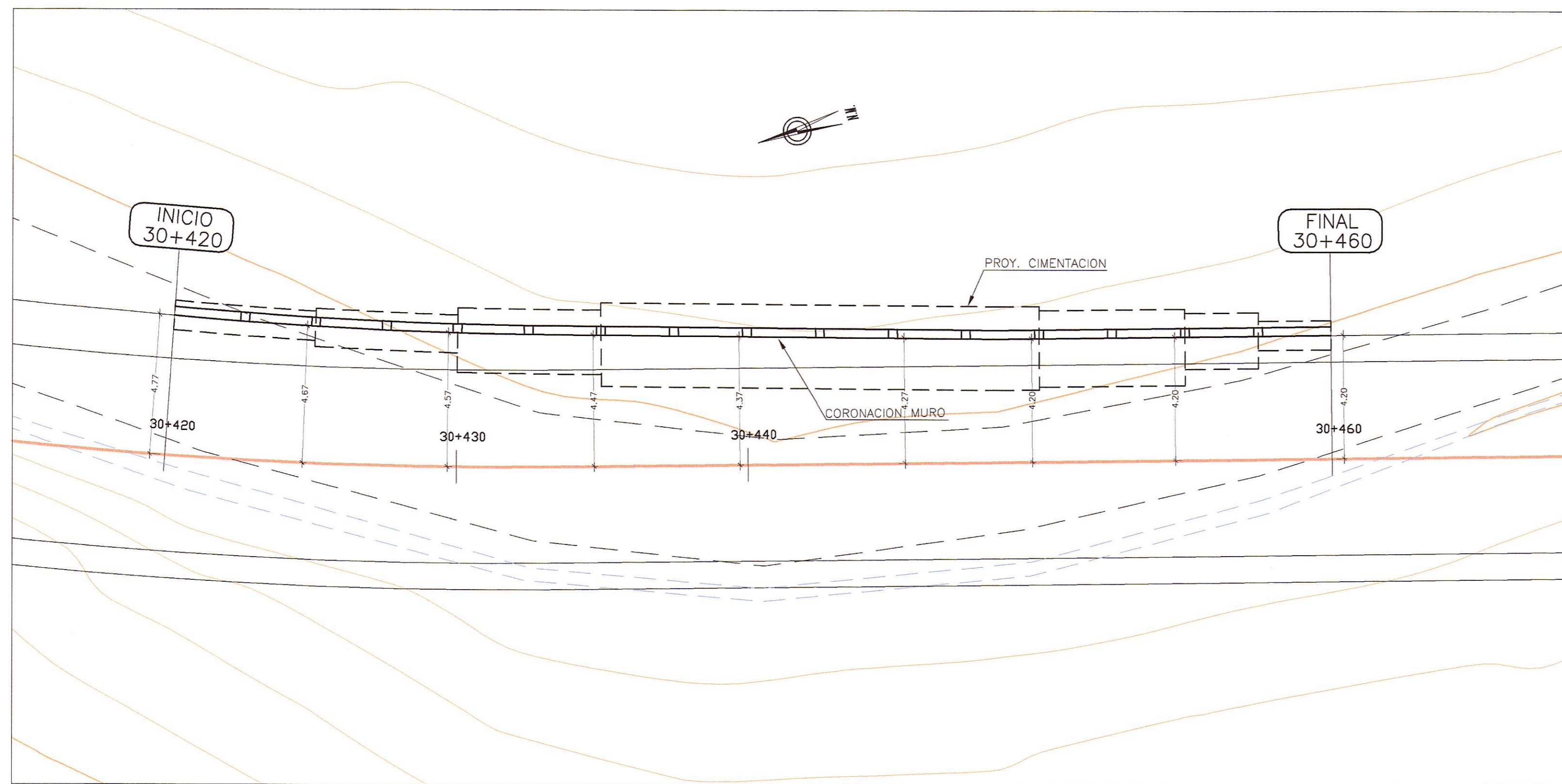
PLANTA ESC. : 1/125
