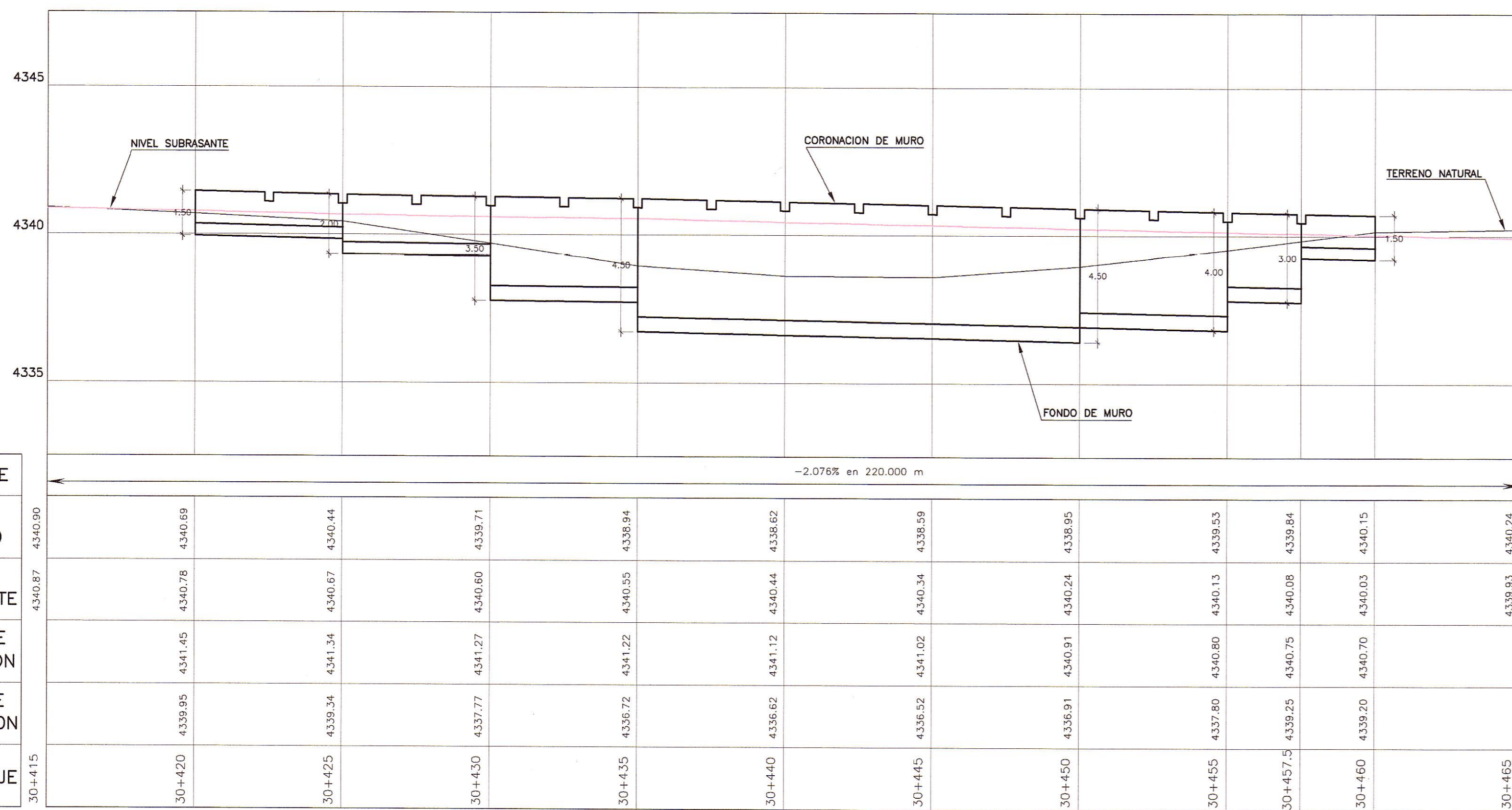
PERFIL LONGITUDINAL
