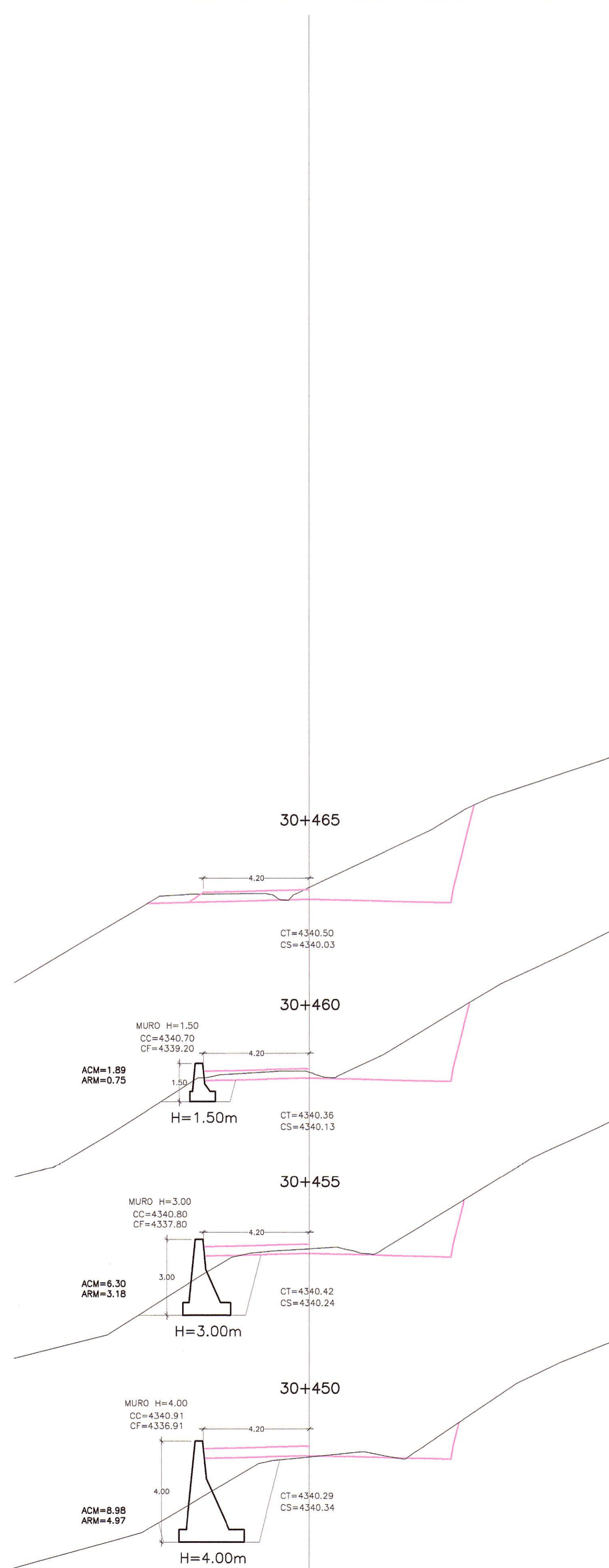
SECCIONES TRANSVERSALES ESC. 1: 1/125
