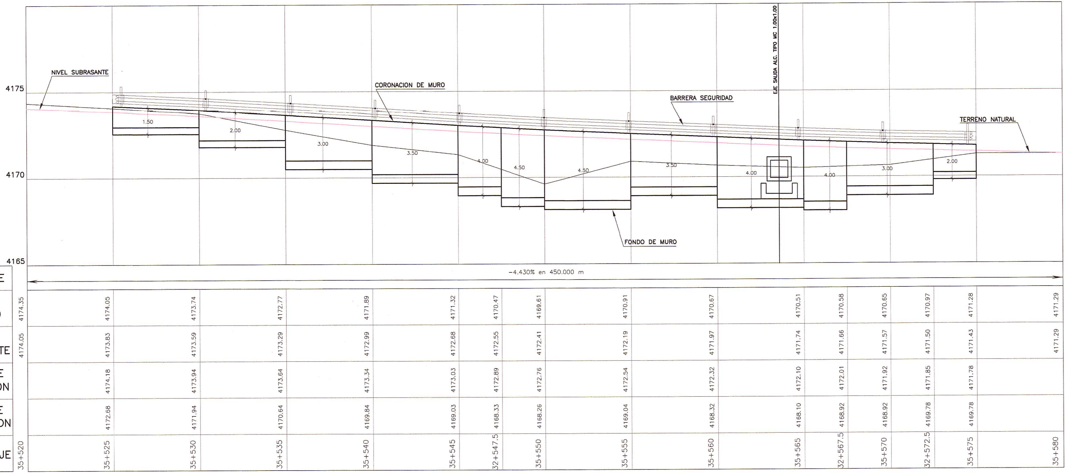
PERFIL LONGITUDINAL ESC. : H=1/125 V=1/125
