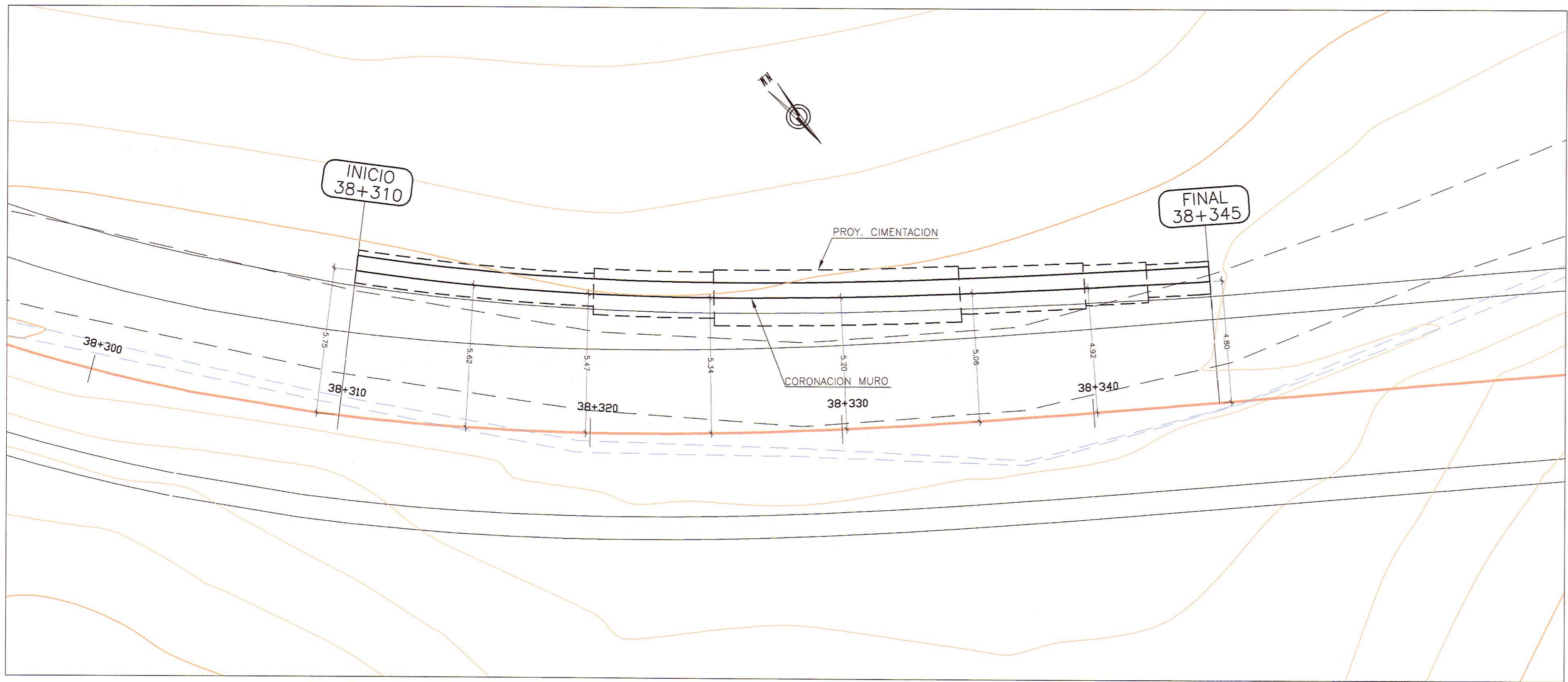
PLANTA ESC.: 1/125
