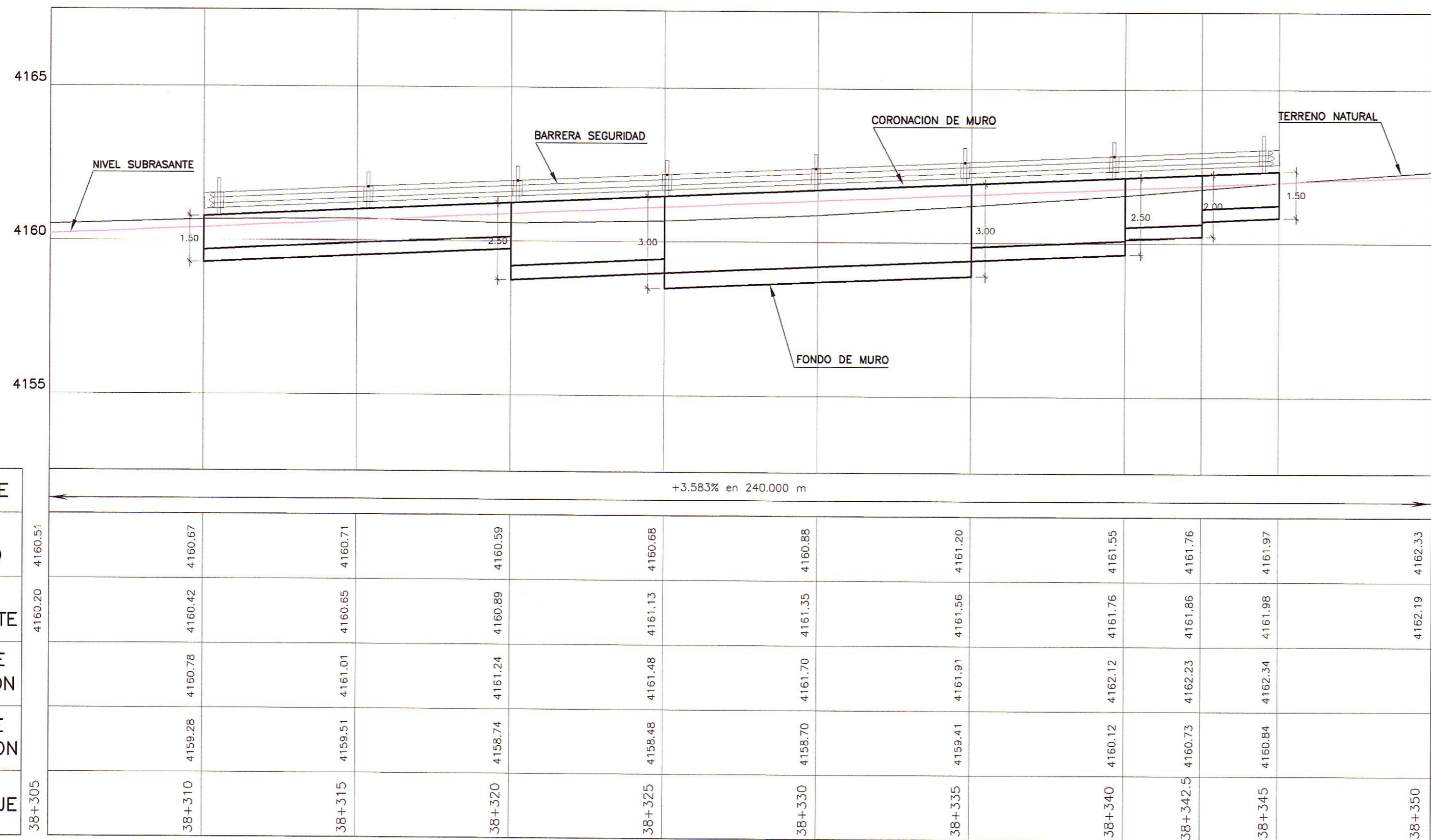
PERFIL LONGITUDINAL
