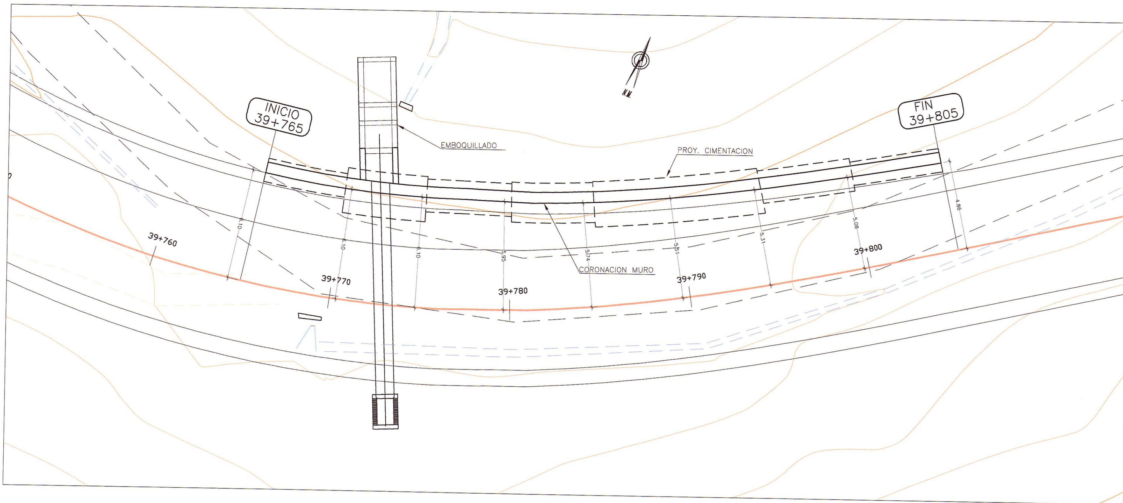
PLANTA ESC. : 1/125
