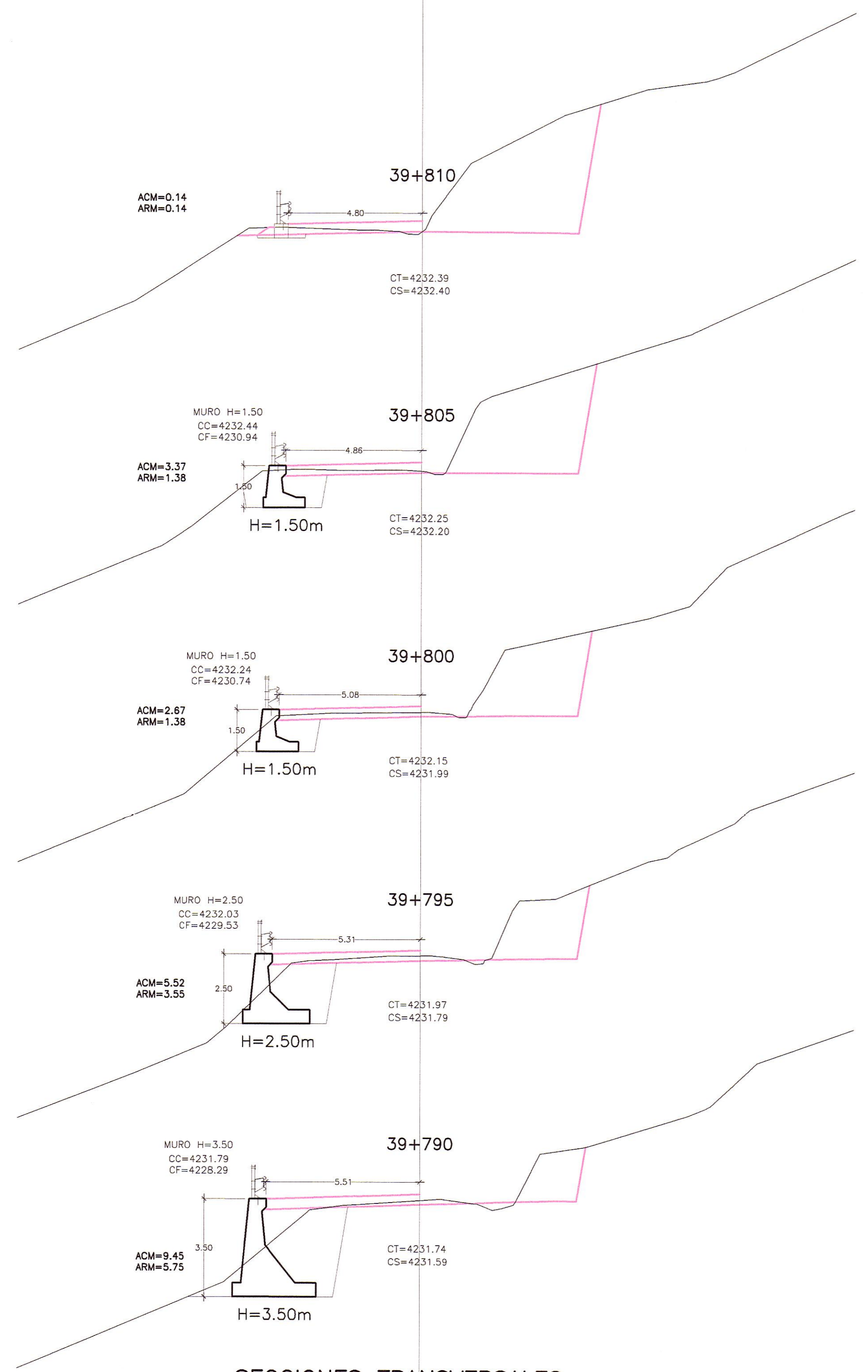
SECCIONES TRANSVERSALES ESC. : 1/125
