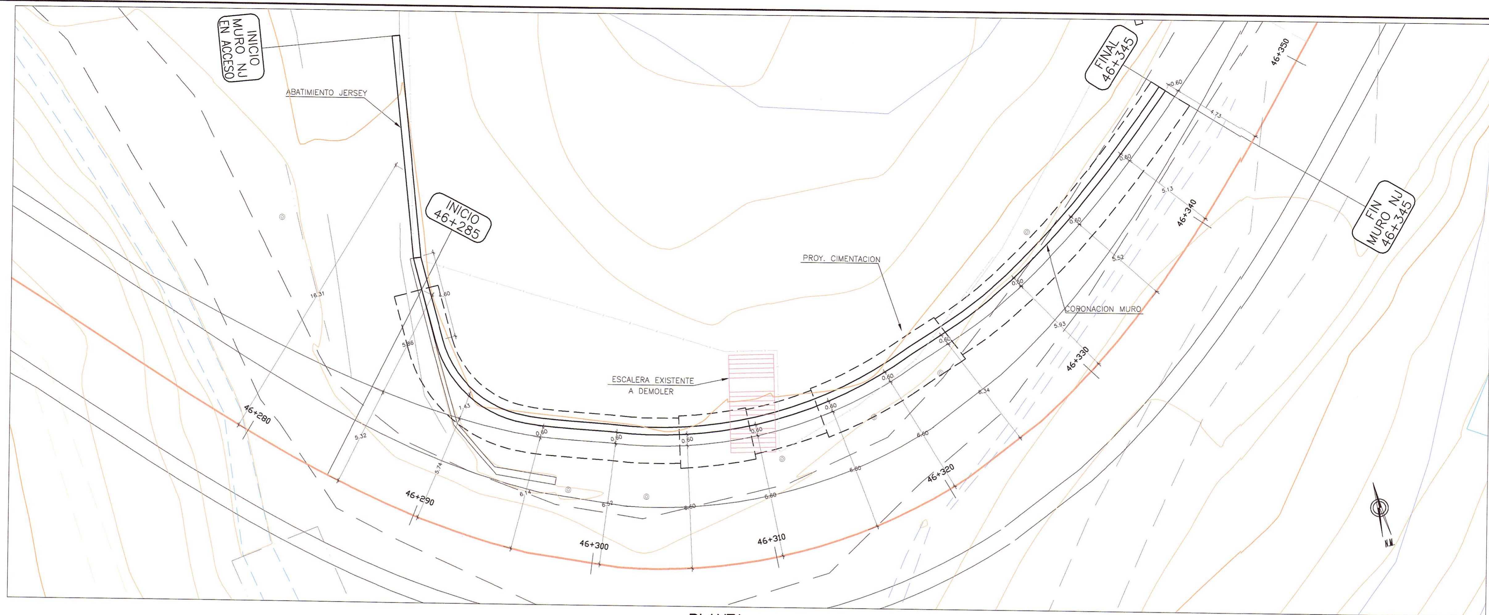
PLANTA ESC. : 1/125
