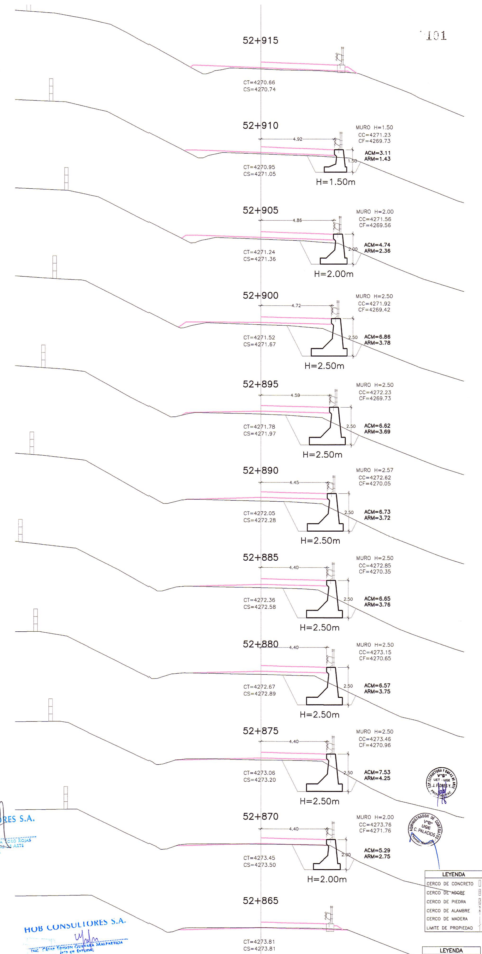
SECCIONES TRANSVERSALES ESC. : 1/125
